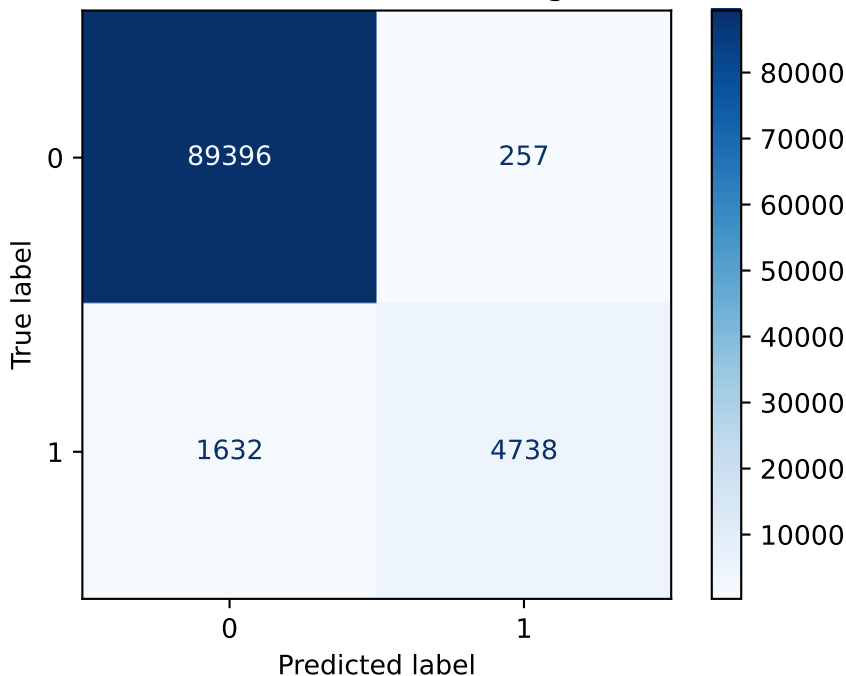
Confusion Matrix: Standard arguments
