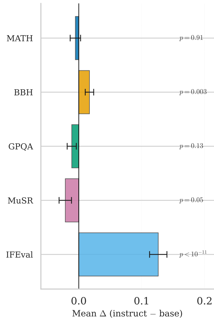
(a) Per-benchmark delta
