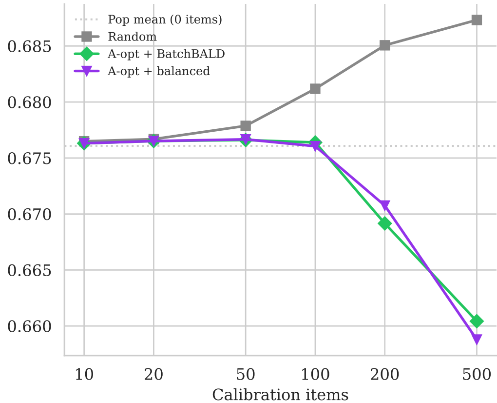
AUC on test items
