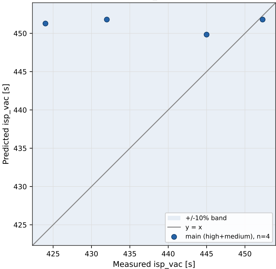
liquid - isp_vac (n=4)
