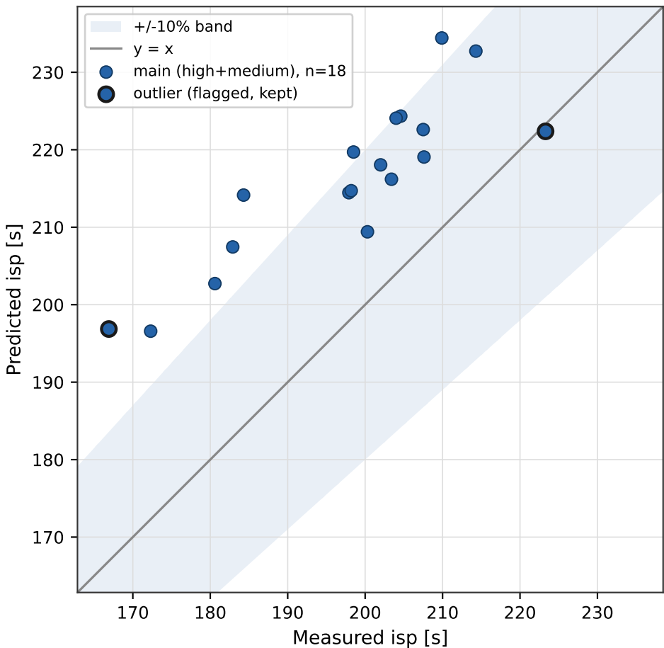
hybrid - isp (n=18)
