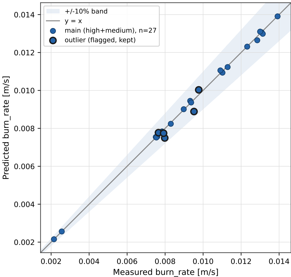
solid - burn_rate (n=27)
