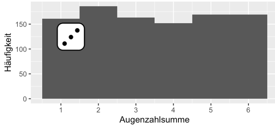
Häufigkeiten von Augenzahlsummen bei 1000 Würfeln
