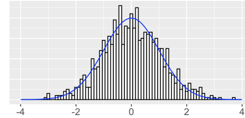
Normalverteilung
