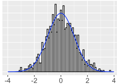
Normalverteilung
