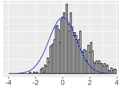
Rechtsschief
