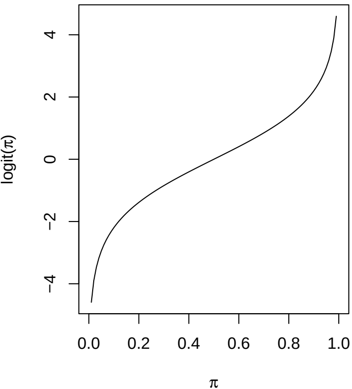
logit-Funktion
