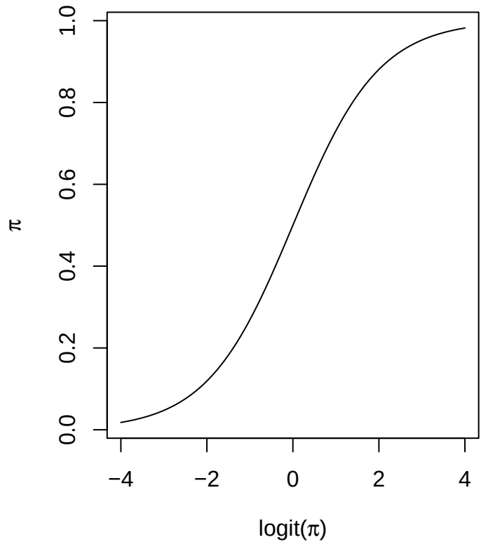
logistische Funktion
