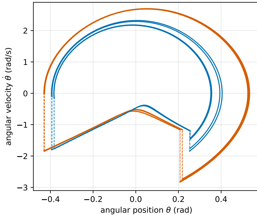
(d) Period 8 | \phi = 5.02^\circ
