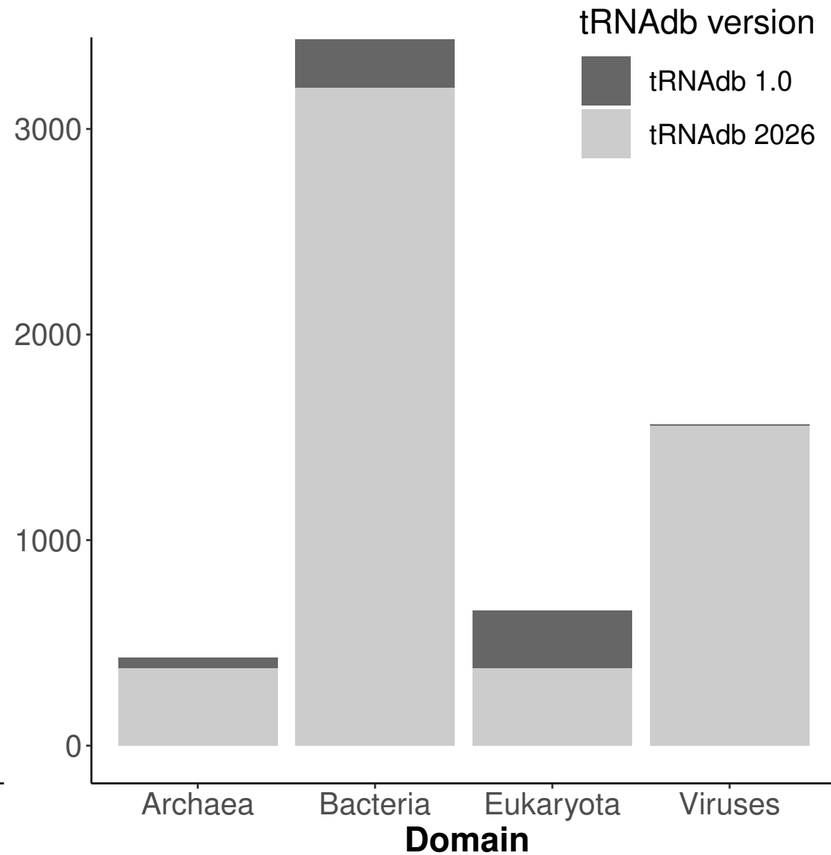
b) genomic tRNAs
