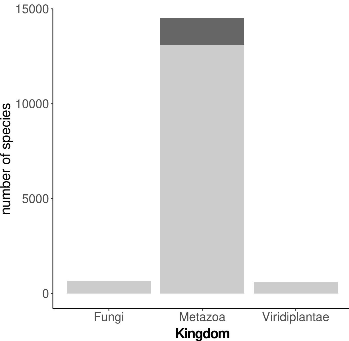
a) mitochondrial tRNAs
