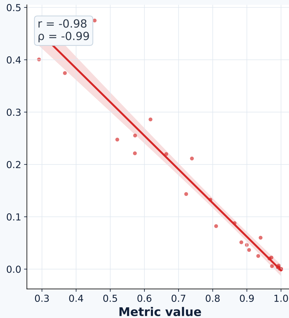
JSD
