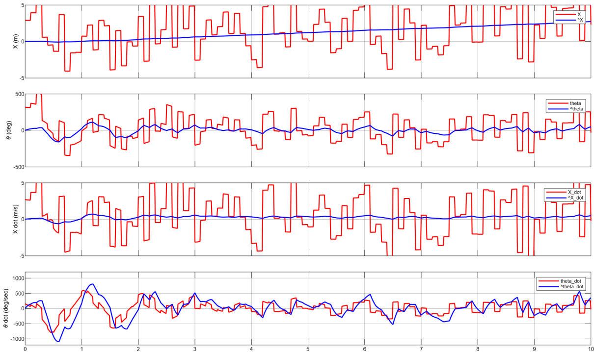
Figura X: Comparació entre l'estat real (vermell) i l'estimació del Filtre de Kalman (blau) per als quatre estats. Cas 5 amb Q_N/R_N = 0.0001 .
