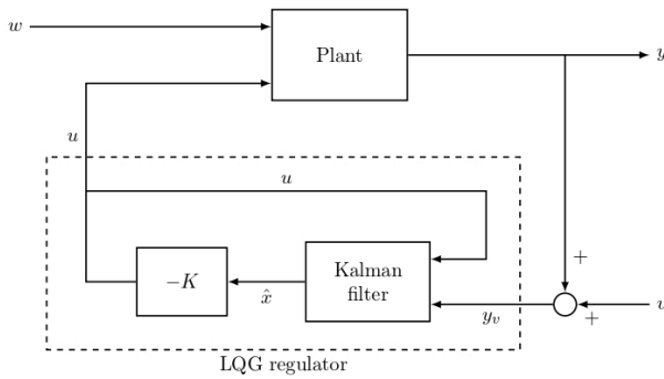
Figura X: Diagrama general del LQG.
