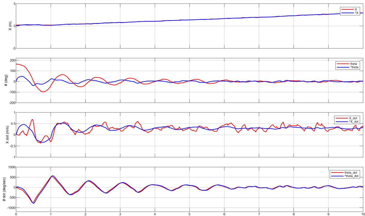
Figura X: Comparació entre l'estat real (vermell) i l'estimació del Filtre de Kalman (blau) per als quatre estats. Cas 2 amb Q_N/R_N = 100 .
