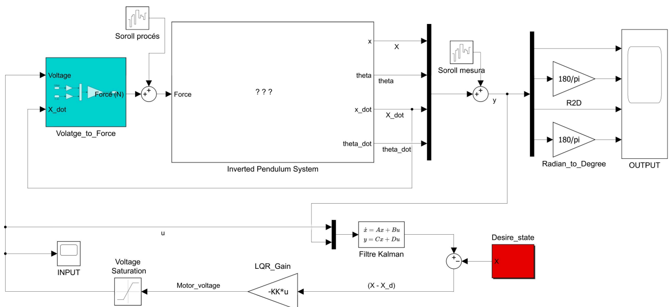
Figura X: Diagrama Simulink del controlador LQG. La planta no lineal rep la força de control generada a partir de l'estimació d'estat multiplicada pel guany LQR. El bloc del Filtre de Kalman reconstrueix els quatre estats a partir de les mesures sorolloses.
