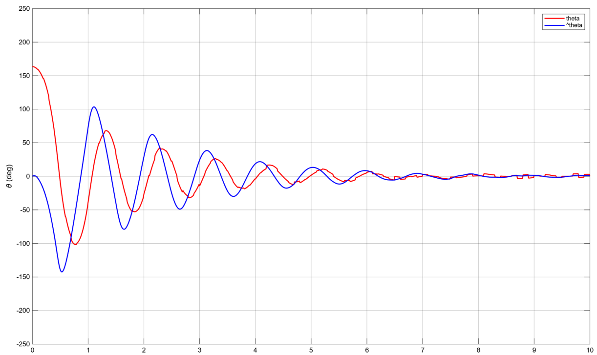
Figura X: Comparació entre l'estat real (vermell) i l'estimació del Filtre de Kalman (blau) per a l'angle del pèndol \theta .
