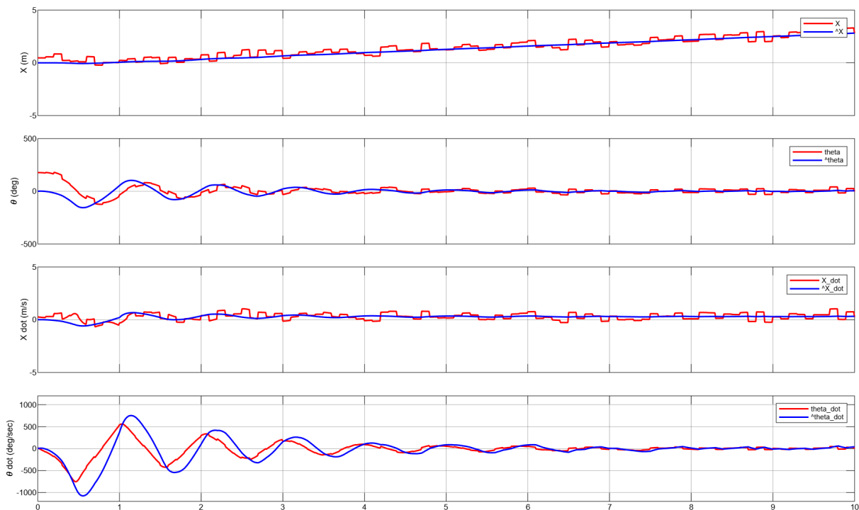
Figura X: Comparació entre l'estat real (vermell) i l'estimació del Filtre de Kalman (blau) per als quatre estats. Cas 3 amb Q_N/R_N = 0.01 .
