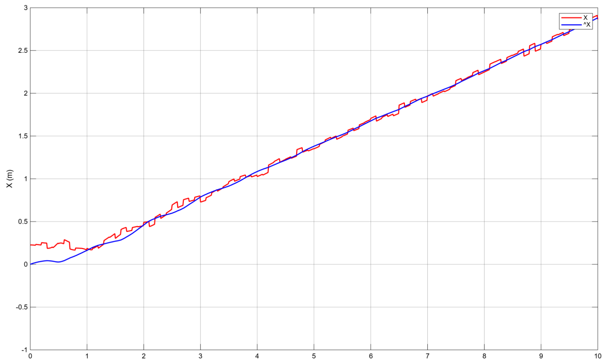
Figura X: Comparació entre l'estat real (vermell) i l'estimació del Filtre de Kalman (blau) per a la posició del carro x .
