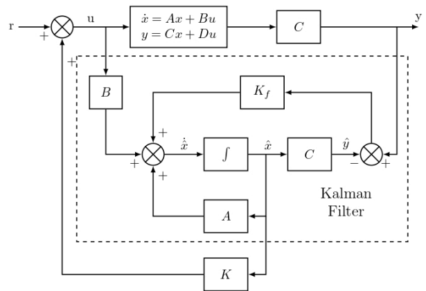
Figura X: Diagrama de blocs detallat del LQG.
