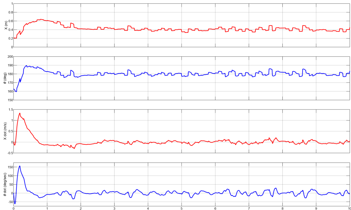
Figura X: Resposta del controlador LQG.
