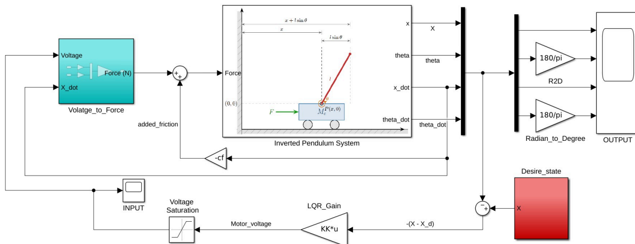
Figura X: Model en Simulink amb fricció addicional.
