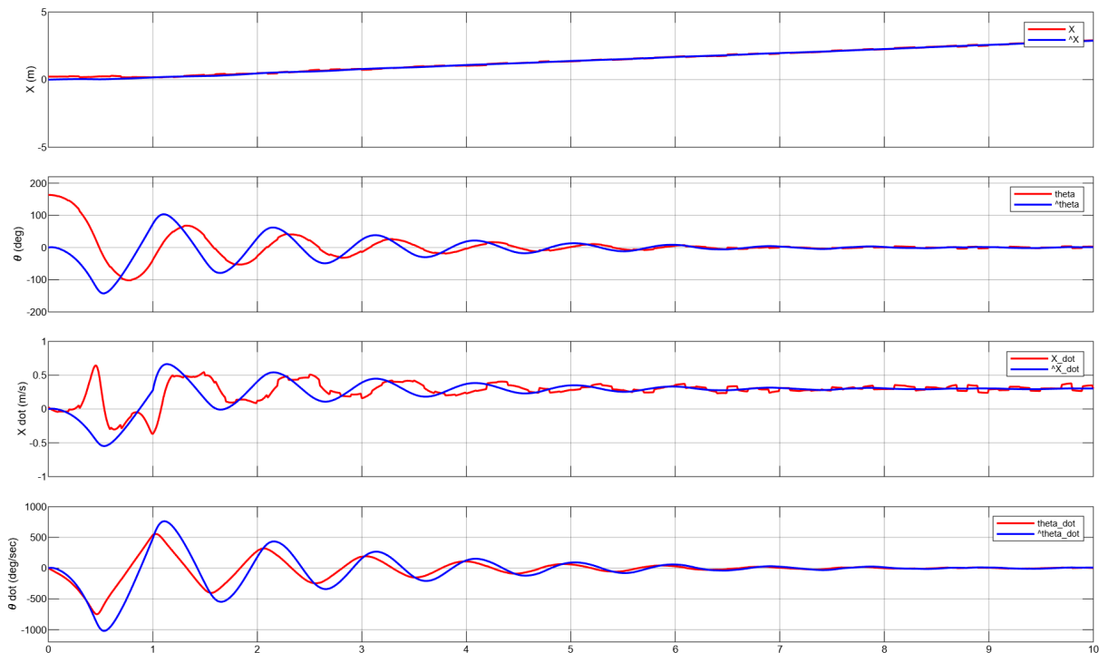
Figura X: Comparació entre l'estat real (vermell) i l'estimació del Filtre de Kalman (blau) per als quatre estats. Cas base amb Q_N = R_N = 0.001 \cdot I_4 .
