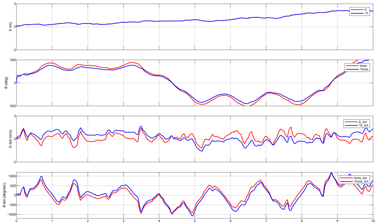
Figura X: Comparació entre l'estat real (vermell) i l'estimació del Filtre de Kalman (blau) per als quatre estats. Cas 4 amb Q_N/R_N = 10\,000 .
