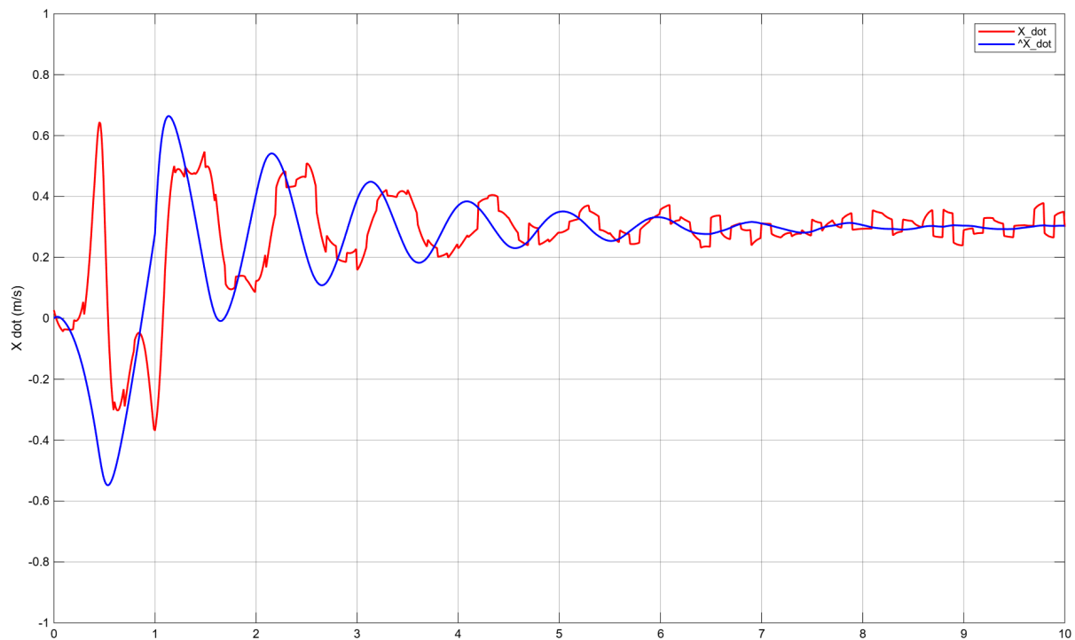
Figura X: Comparació entre l'estat real (vermell) i l'estimació del Filtre de Kalman (blau) per a la velocitat del carro \dot{x} .
