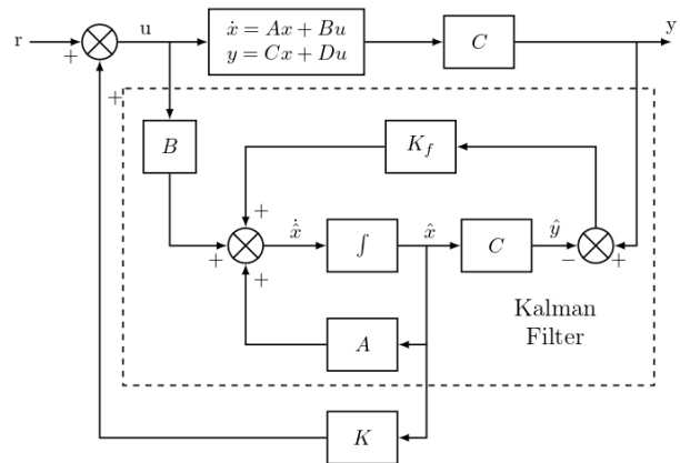
Figura 19: Diagrama de blocs detallat del LQG.
