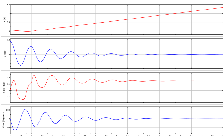
Figura 3: Resposta del sistema en llaç obert a un esglaó de tensió de 1V.
