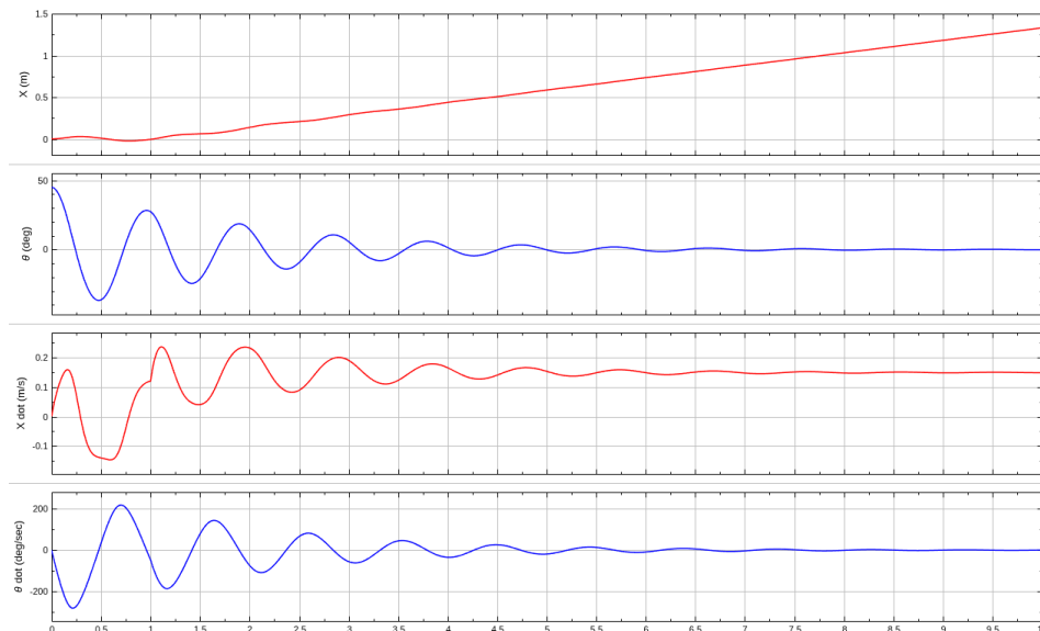
Figura X: Resposta del sistema en llaç obert a un esglao de tensió de 1V.
