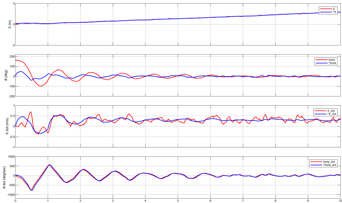
Figura 36: Comparació entre l'estat real (vermell) i l'estimació del Filtre de Kalman (blau) per als quatre estats. Cas 2 amb Q\_N/R\_N = 100 .
