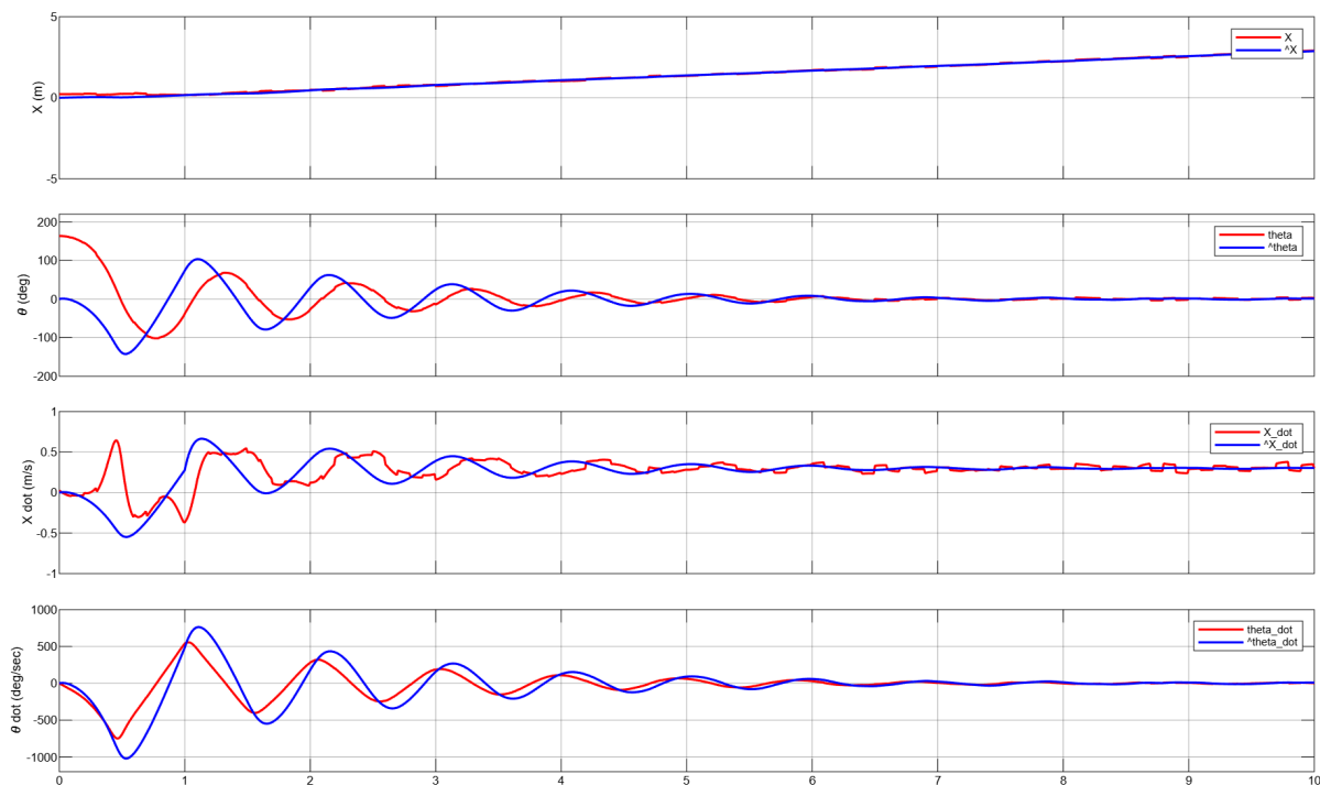
Figura 35: Comparació entre l'estat real (vermell) i l'estimació del Filtre de Kalman (blau) per als quatre estats. Cas base amb Q_N = R_N = 0.001 \cdot I_4 .
