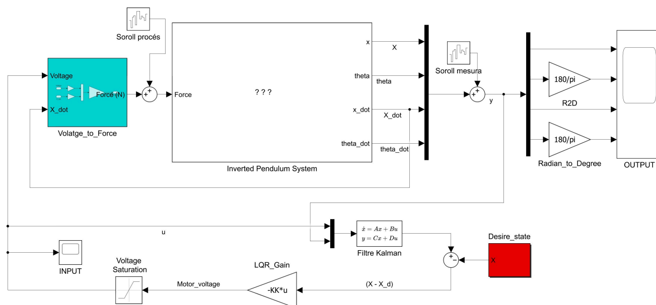
Figura 20: Diagrama Simulink del controlador LQG. La planta no lineal rep la força de control generada a partir de l'estimació d'estat multiplicada pel guany LQR. El bloc del Filtre de Kalman reconstrueix els quatre estats a partir de les mesures sorolloses.
