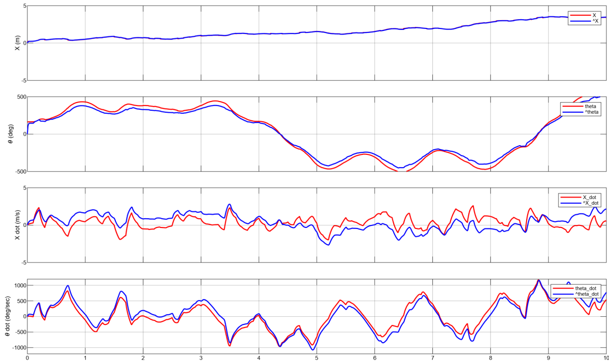
Figura 38: Comparació entre l'estat real (vermell) i l'estimació del Filtre de Kalman (blau) per als quatre estats. Cas 4 amb Q_N/R_N = 10\,000 .
