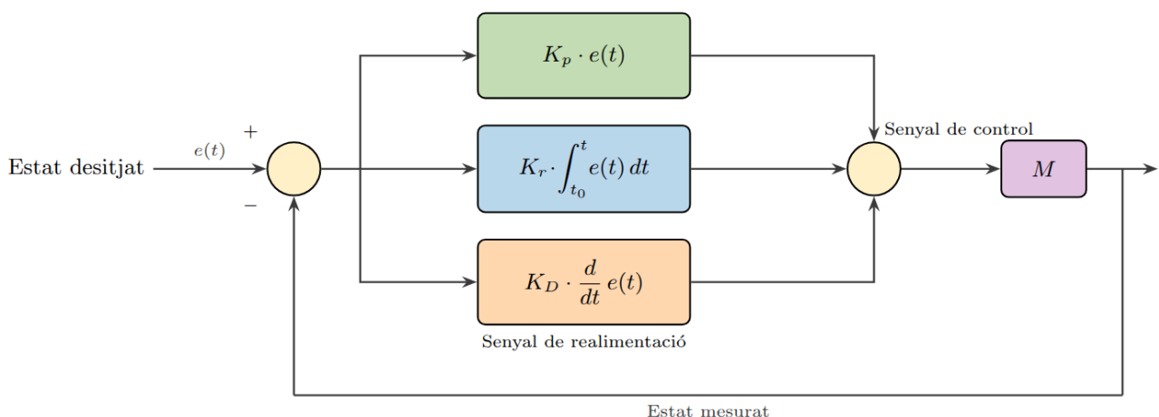
Figura 4: Esquema bàsic d'un controlador PID.
