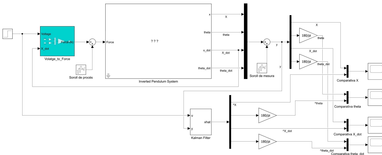
Figura 13: Diagrama Simulink de l'estimació d'estat amb el Filtre de Kalman. La planta no lineal rep com a entrada la força generada pel subsistema Voltage_to_Force . Les sortides s'afegeix soroll de mesura i de procés i s'introdueix al bloc Kalman Filter , que reconstrueix els quatre estats estimats del sistema.
