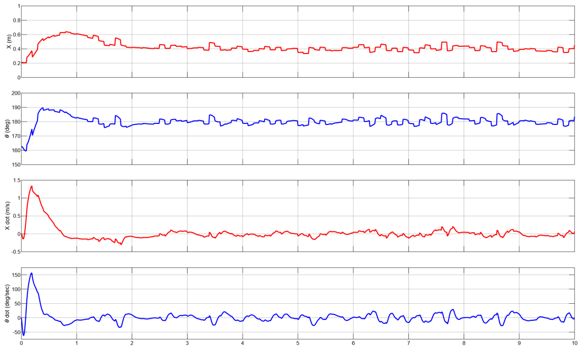
Figura 21: Resposta del controlador LQG.
