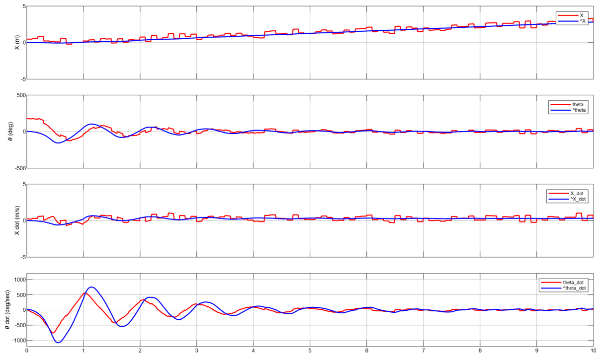
Figura 37: Comparació entre l'estat real (vermell) i l'estimació del Filtre de Kalman (blau) per als quatre estats. Cas 3 amb Q\_N/R\_N = 0.01 .
