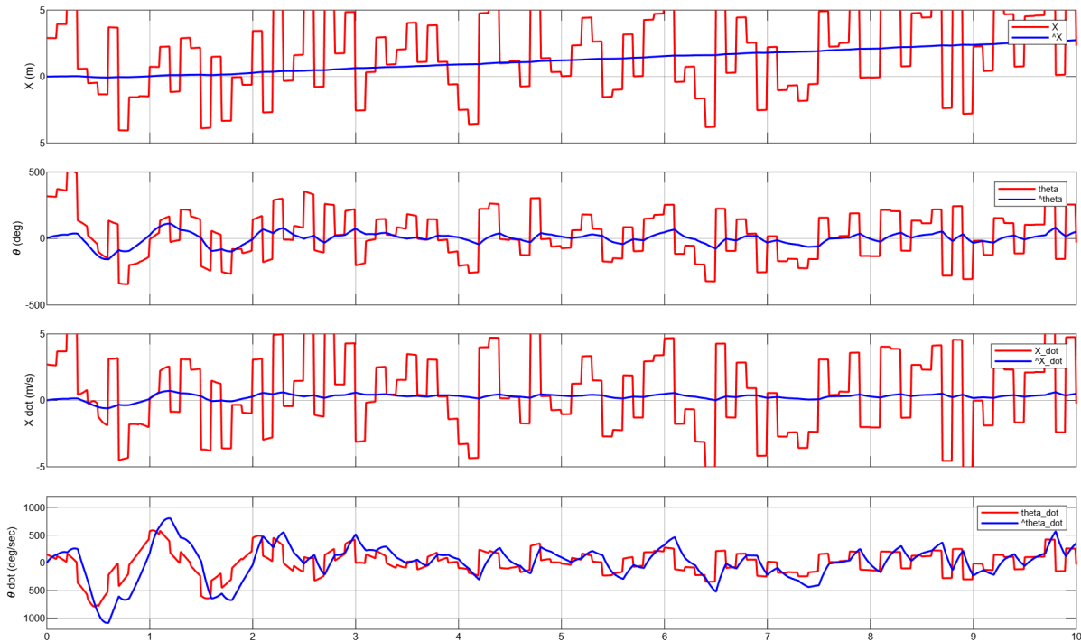
Figura 39: Comparació entre l'estat real (vermell) i l'estimació del Filtre de Kalman (blau) per als quatre estats. Cas 5 amb Q_N/R_N = 0.0001 .
