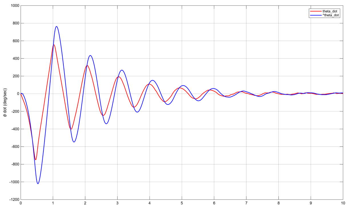
Figura 17: Comparació entre l'estat real (vermell) i l'estimació del Filtre de Kalman (blau) per a la velocitat angular del pèndol.
