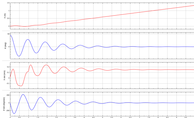
Figura X: Resposta del sistema en llaç obert a un esglaó de tensió de 1V.
