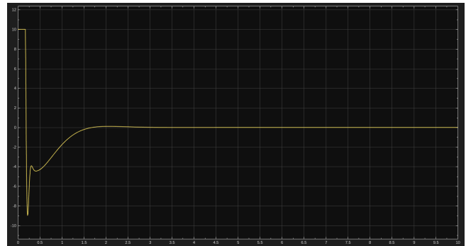
Figura X: Voltatge del sistema amb fricció addicional elevada
