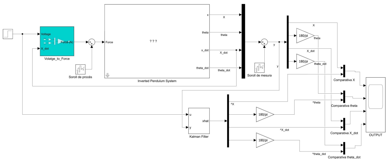
Figura X: Diagrama Simulink de l'estimació d'estat amb el Filtre de Kalman. La planta no lineal rep com a entrada la força generada pel subsistema Voltage_to_Force . Les sortides s'afegeix soroll de mesura i de procés i s'introdueix al bloc Kalman Filter , que reconstrueix els quatre estats estimats \hat{x} , \hat{\theta} , \hat{\dot{x}} i \hat{\dot{\theta}} .
