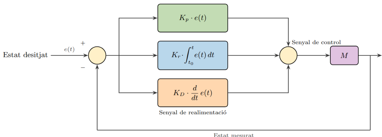
Figura X: Esquema bàsic d'un controlador PID.
