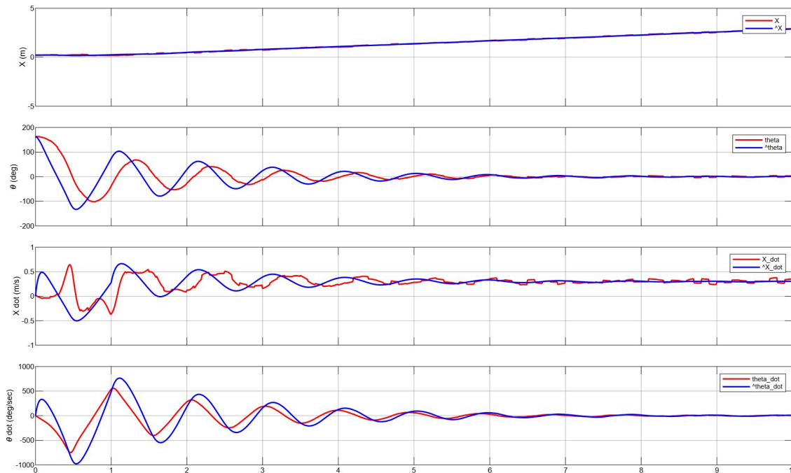
Figura X: Comparació entre l'estat real (vermell) i l'estimació del Filtre de Kalman (blau) per als quatre estats del sistema: posició del carro x , angle del pèndol \theta , velocitat del carro \dot{x} i velocitat angular del pèndol \dot{\theta} . Simulació de 10 s amb condicions inicials x_0 = [0.2, \pi - 0.1\pi, 0, 0]^T i soroll de procés i de mesura amb covariància Q = 0.001I_4 .
