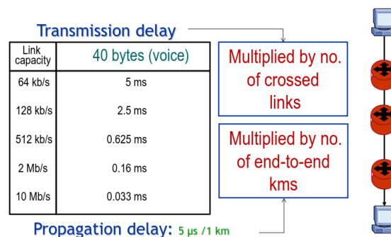
Figure 6.6: Ritardo da trasmissione e propagazione
