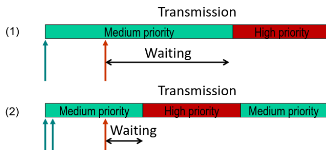
Figure 5.6: Effetto di un pacchetto lungo a priorità media
