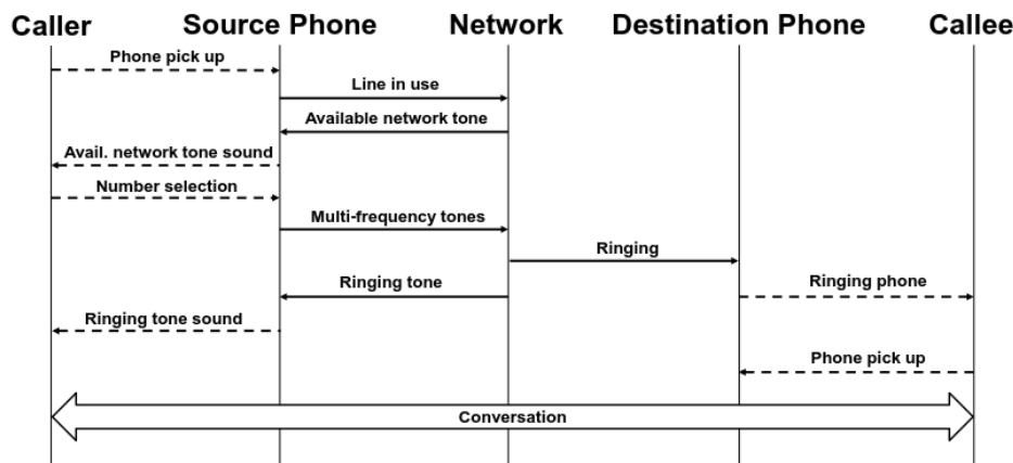
Figure 6.9: Diagramma di sequenza di SS7
