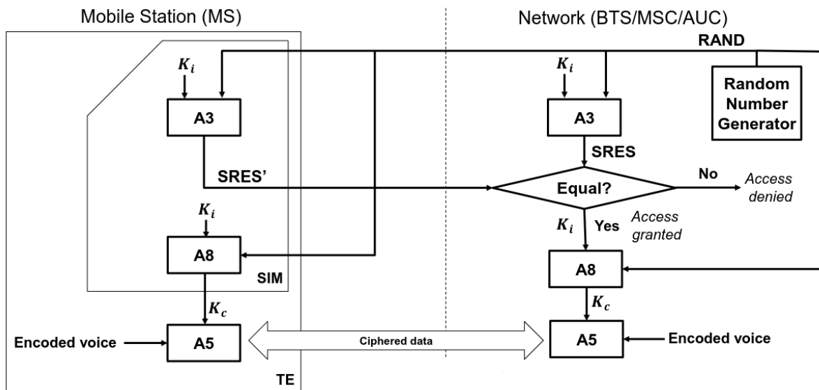
Figure 9.4: Autenticazione e cifratura in GSM
