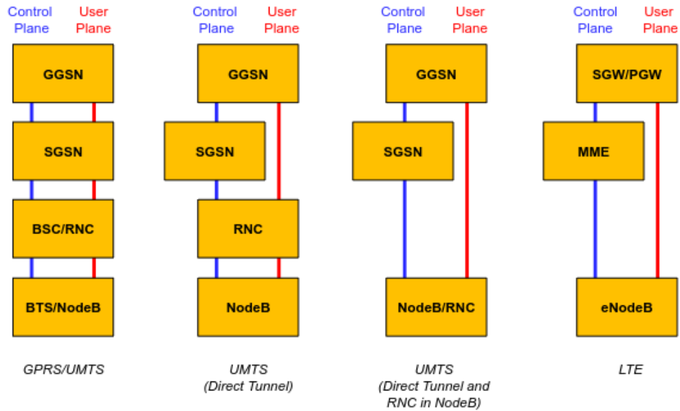
Figure 11.2: Evoluzione delle reti mobili verso un'architettura flat
