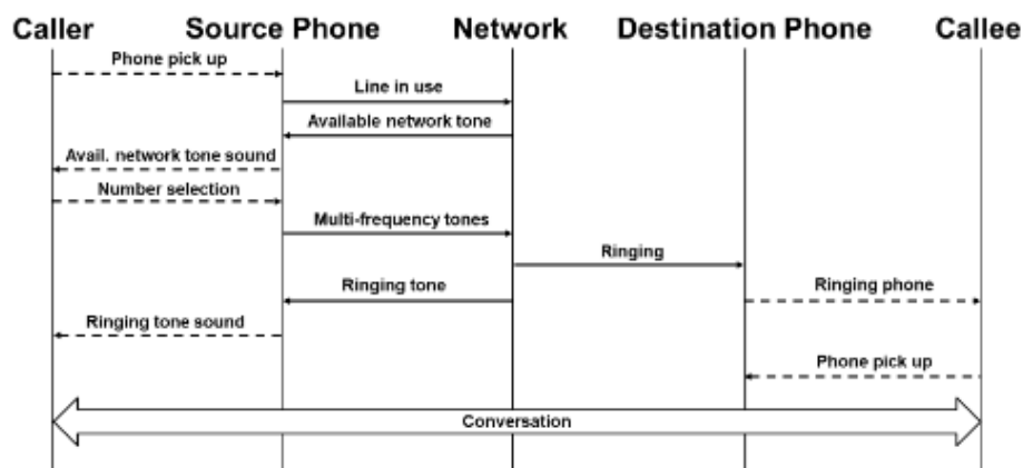
Figure 9.10: Chiamata iniziata dalla MS
