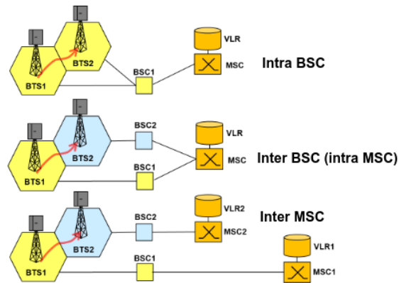
Figure 9.14: Tipi di handover in GSM
