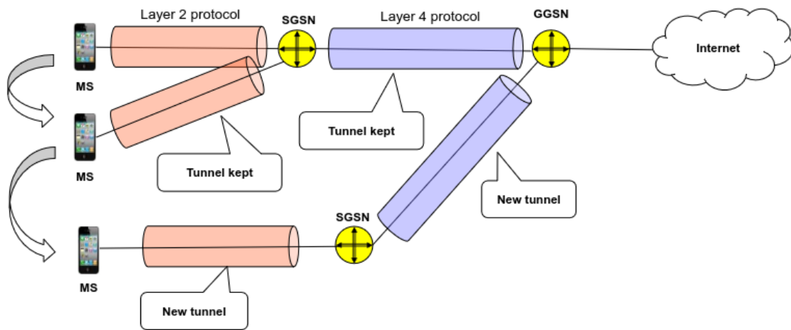
Figure 9.18: Tunneling e mobilità in GPRS/EDGE
