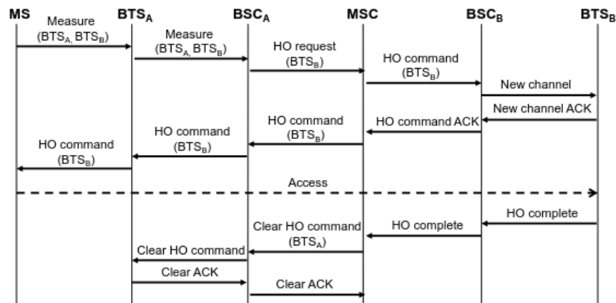
Figure 9.15: Diagramma di sequenza per handover in GSM
