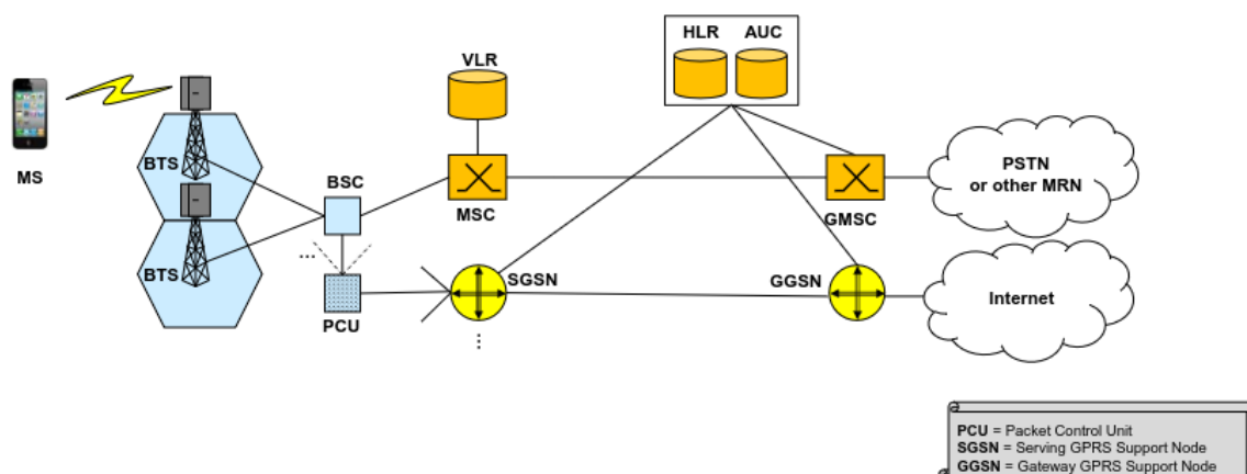
Figure 9.16: Architettura di rete EDGE
