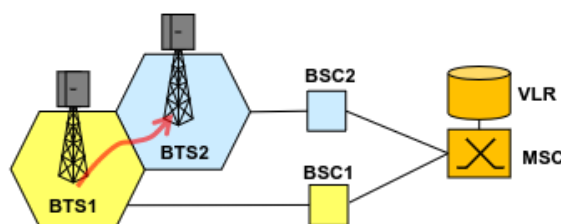
Figure 9.6: Location update tra due LA servite dallo stesso MSC/VLR
