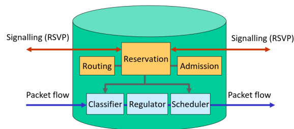
Figure 5.7: Funzionalità dei router in IntServ
