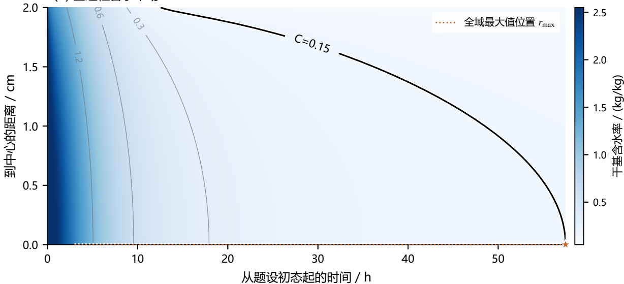
(b) 全过程含水率场
