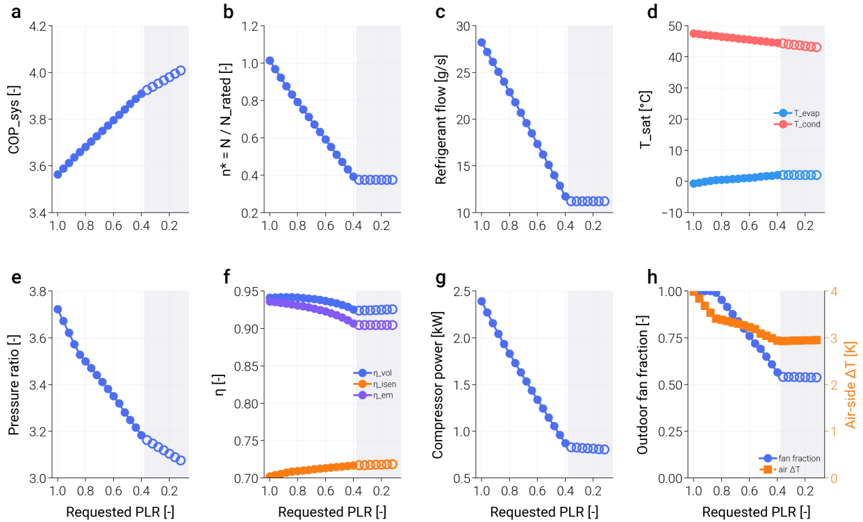
그림 8: F8a. 공기→물 9 kW R32, 외기 7 °C / 탱크 42.5 °C — 요구 PLR에 따른 내부 상태(속 빈 마커 = 속도 하한, 공급 > 요구)
