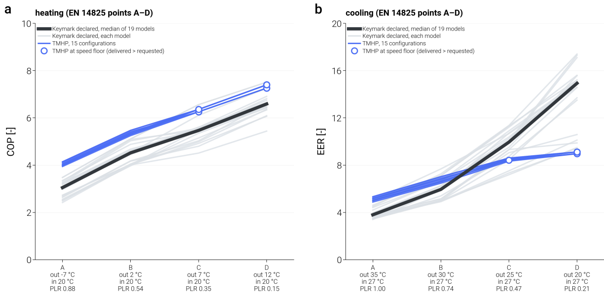
그림 10: F10. 공기→공기 EN 14825 궤적 — 모델 15 구성 vs Keymark 선언 19 모델(회색), 중앙값(검정). 각 점의 외기·실내 온도와 부분부하율을 눈금 아래에 적었다
