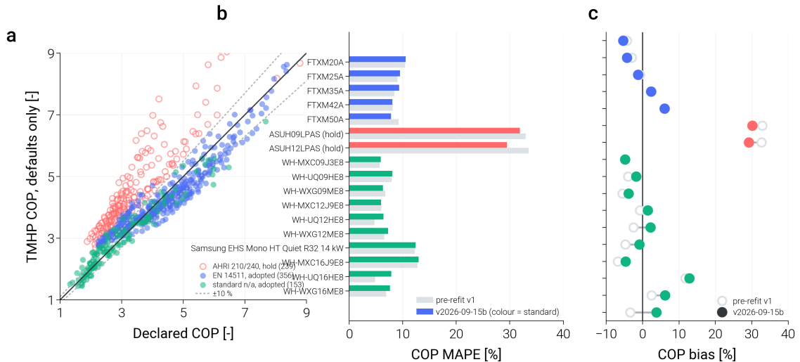
그림 7: F7. 카탈로그 패리티 — 계수 동결, 정격규격·상태별 증화, 기기별 구(v1)·신(v2026-09-15b) 비교
