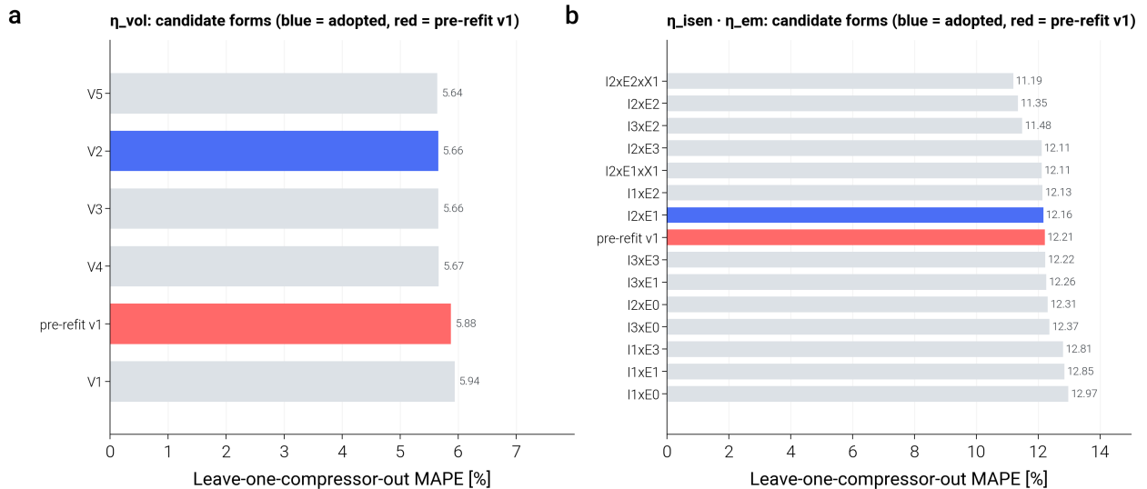
그림 5: F5. 후보 식의 LOCO 가중 MAPE
