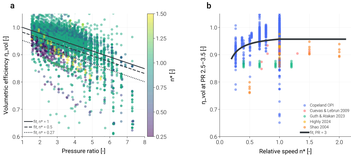
그림 2: F2. 체적효율 — 데이터와 채택식 V2
