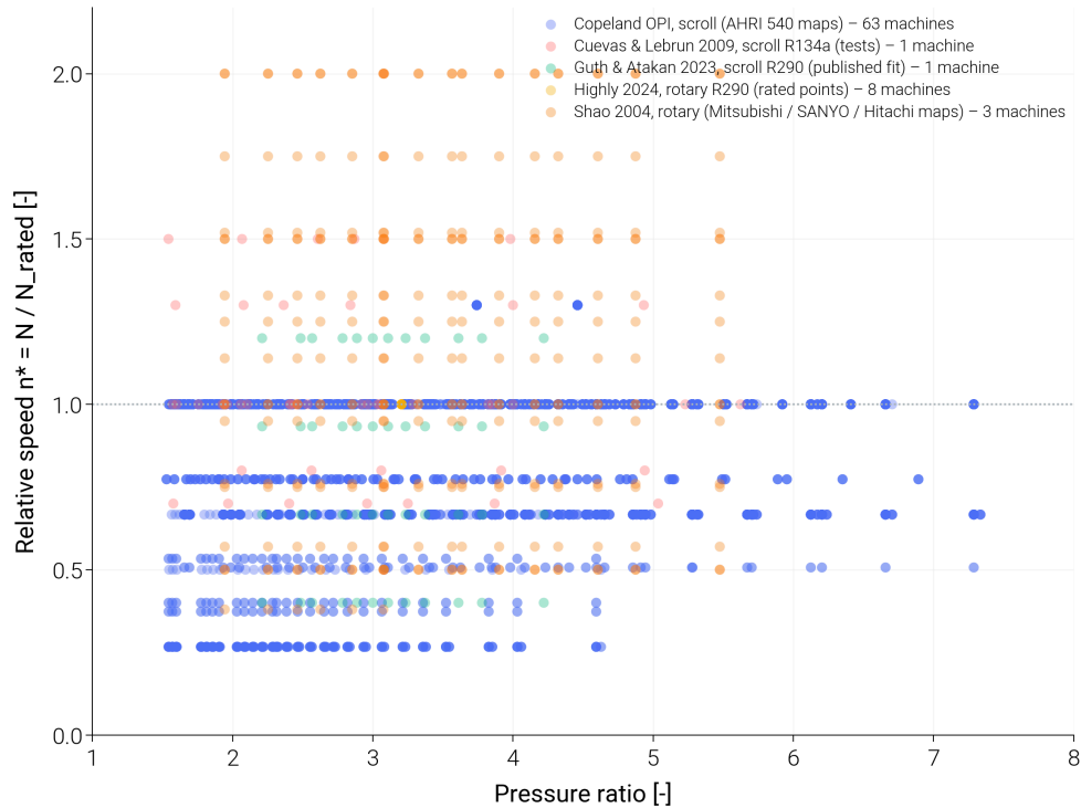
그림 1: F1. 적합에 쓰인 압축기 데이터의 PR × n* 범위
