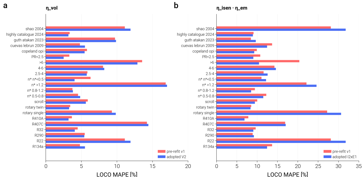
그림 6: F6. 층별 LOCO 오차 — 채택식 vs 구 기본값
