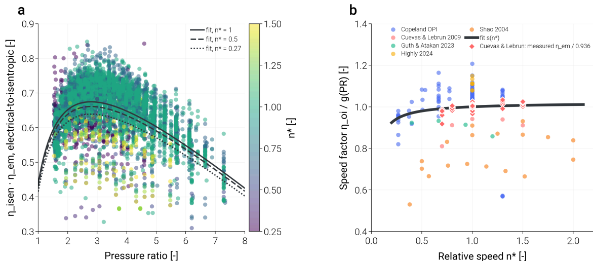
그림 3: F3. 전기→등엔트로피 곱 g(PR) \cdot s(n^*) 와 속도 인자의 소스별 증거
