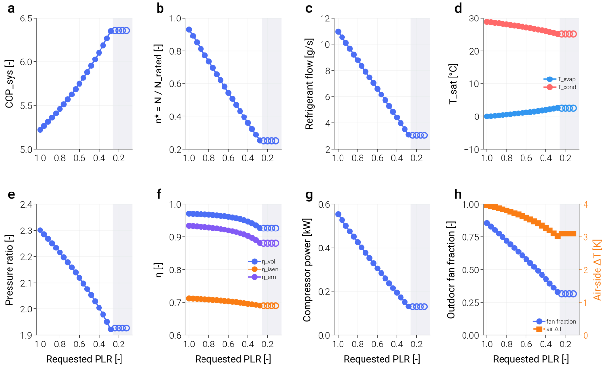
그림 9: F8b. 공기→공기 3.5 kW R32 난방, 외기 7 °C / 실내 20 °C
