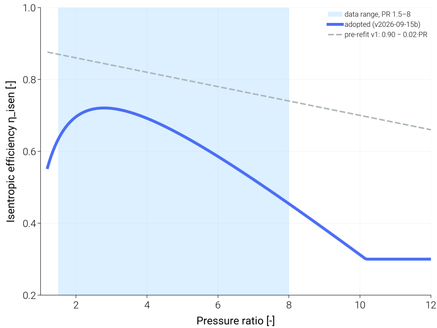
그림 4: F4. 등엔트로피 효율 — 채택식과 구 선형식
