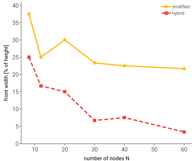
numerical diffusion vs N
