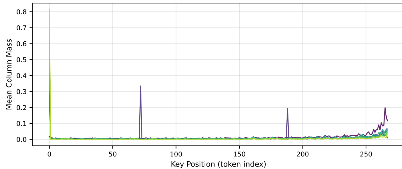
Qwen3-8B (en)
