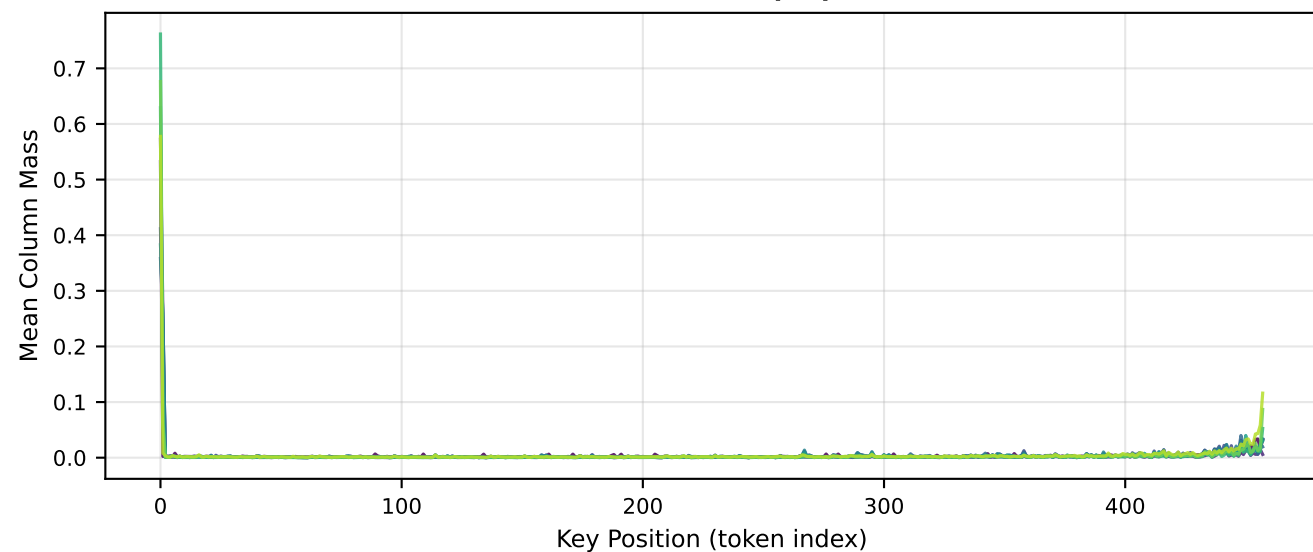
Qwen3-4B (zh)
