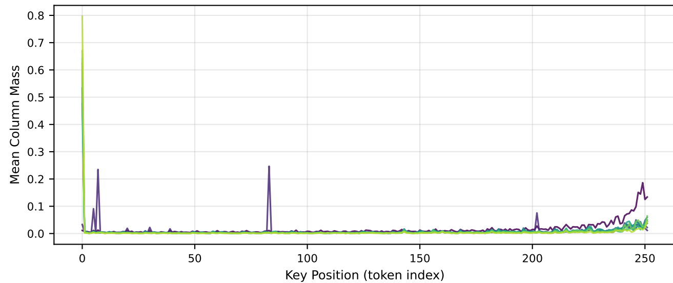
Qwen3-8B (zh)
