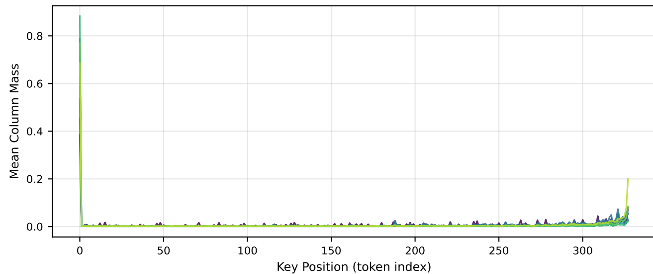
Mistral-7B (zh)
