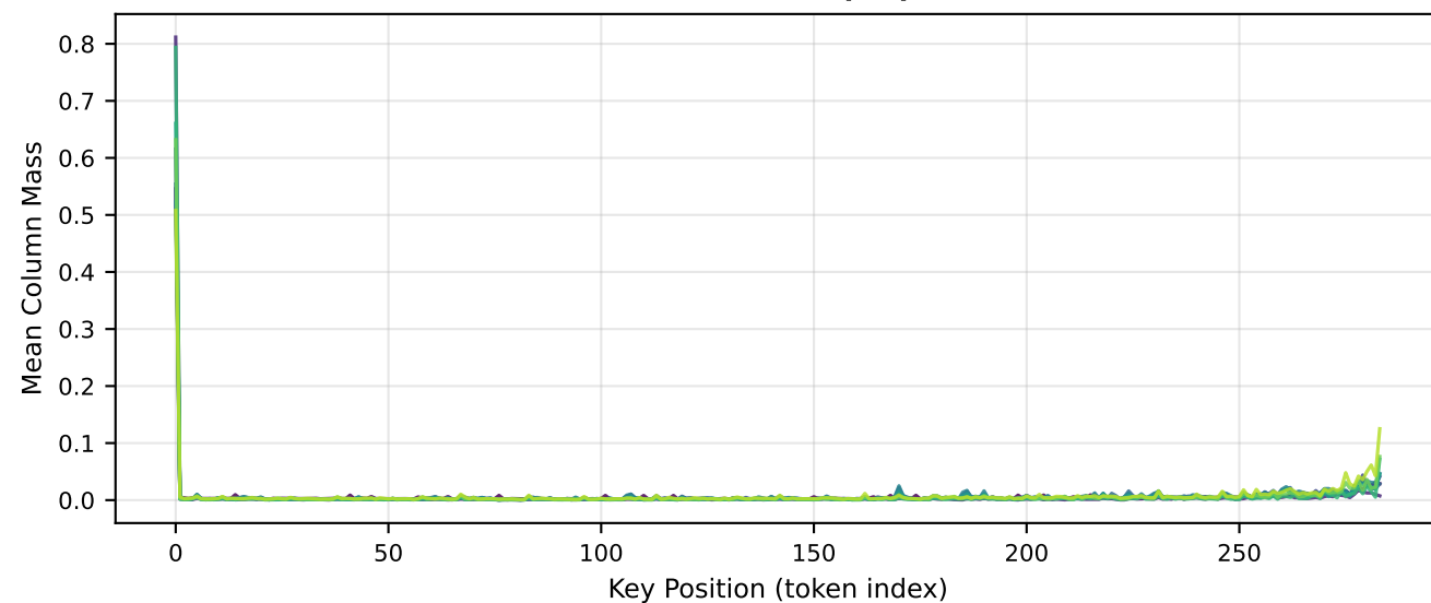
Qwen3-4B (en)
