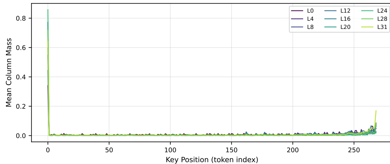
Mistral-7B (en)
