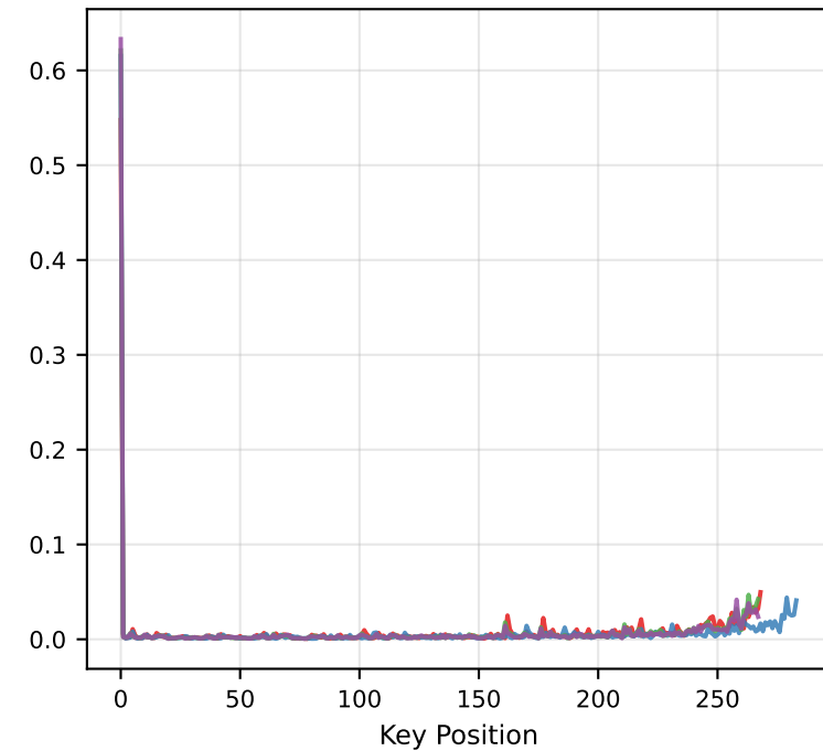
Layer 8
