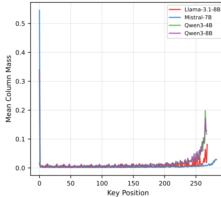
Layer 0
