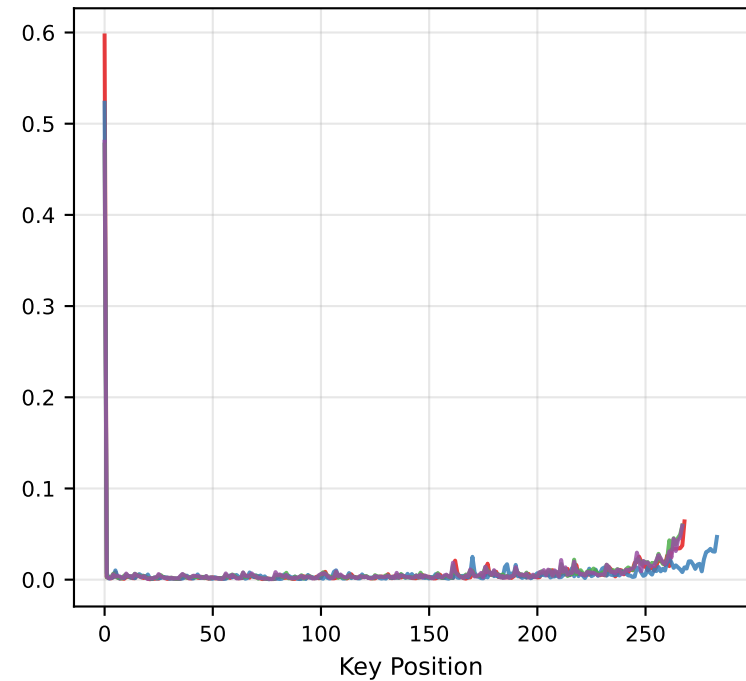
Layer 16
