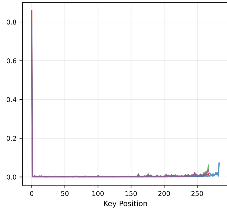
Layer 24
