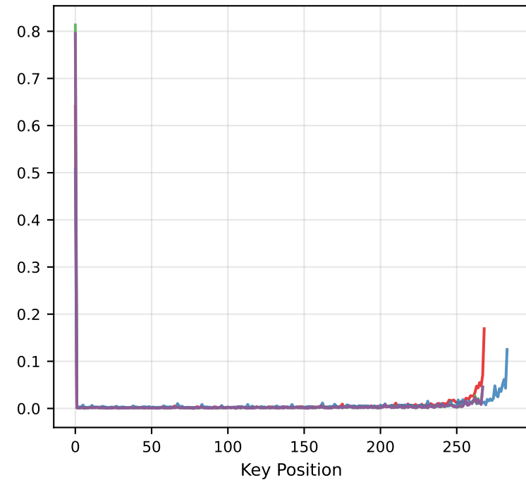
Layer 31
