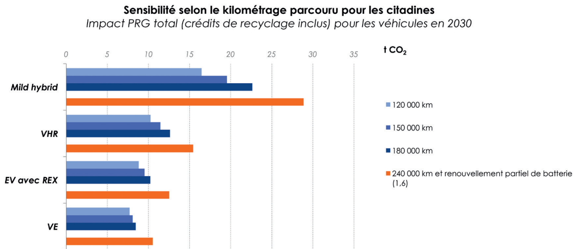
Figure 33 : Sensibilité au kilométrage parcouru en 10 ans pour les citadines et berlines électriques
