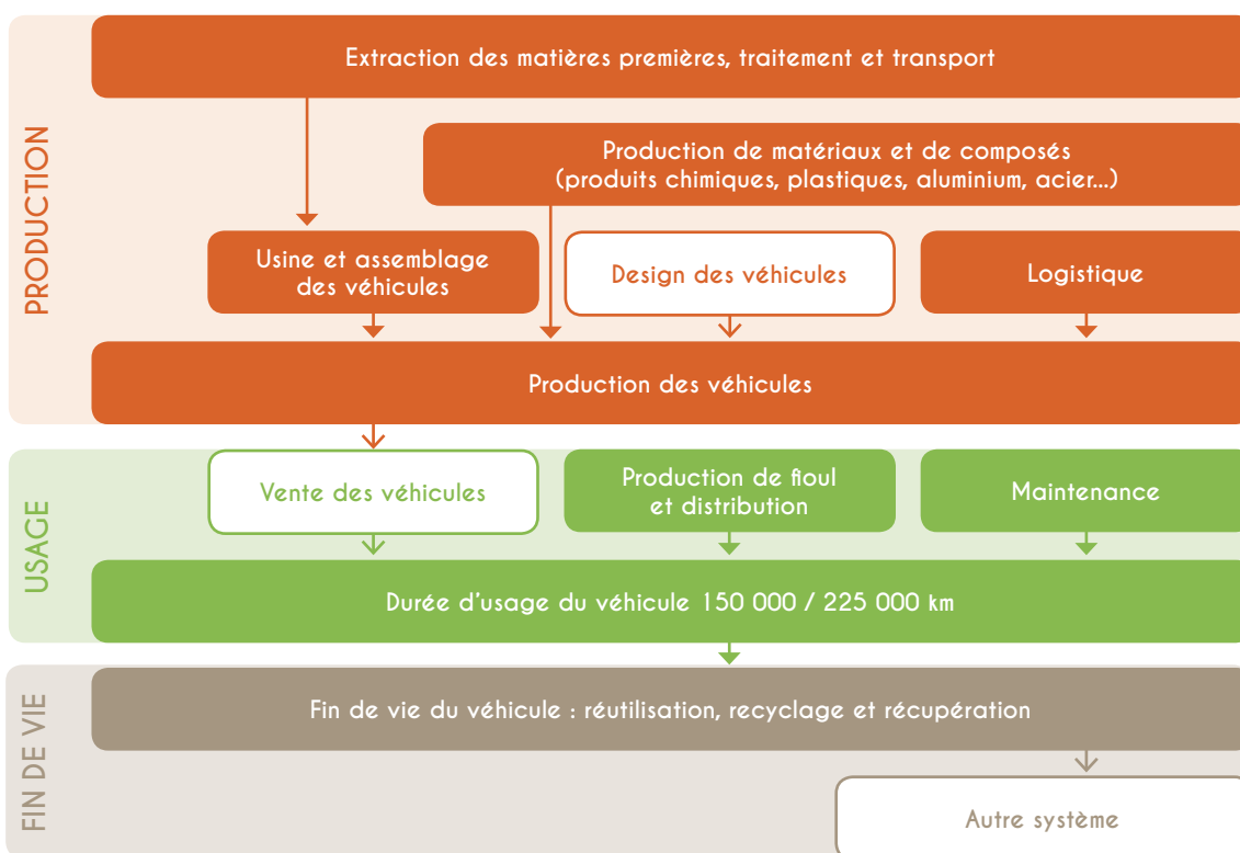
Figure 4 : Périmètre de l'analyse de cycle de vie (ACV)
