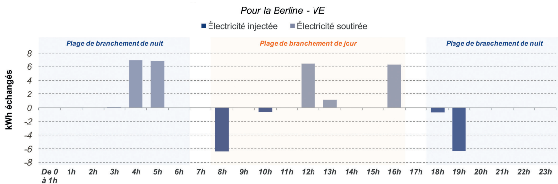
Figure 18 : Echanges d'électricité avec le véhicule en V2G
