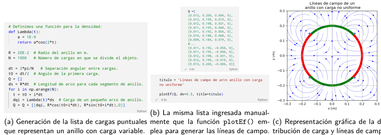
Figura 8: Cálculo de líneas de campo eléctrico generadas por una distribución de carga en un anillo.
