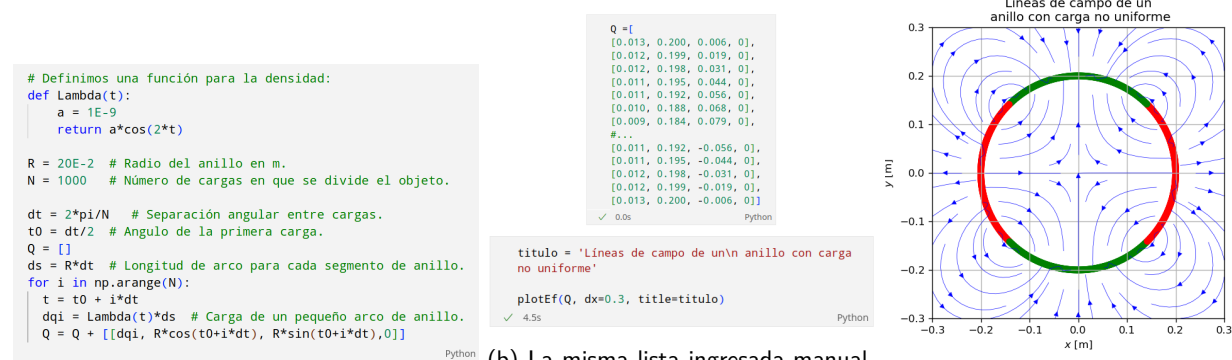
Figura 8: Cálculo de líneas de campo eléctrico generadas por una distribución de carga en un anillo.
