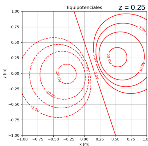
»'''Figura 8: Con una simple línea de código se pueden estudiar las curvas equipotenciales resultantes de la intersección de las superficies equipotenciales con planos a diferentes alturas ( z = 0 , z = 0,25 y z = 0,5 ) respecto »'''de las cargas.
