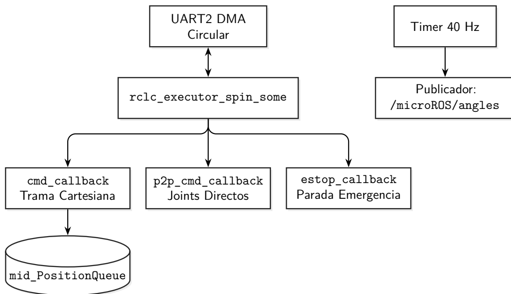
Figura 3.3: Diagrama de bloques Firmware Detalle 1: defaultTask y micro-ROS.
