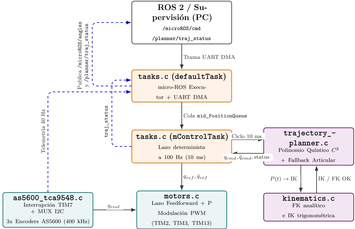
Figura 3.1: Mapa de interacción y acoplamiento funcional de los módulos del firmware.
