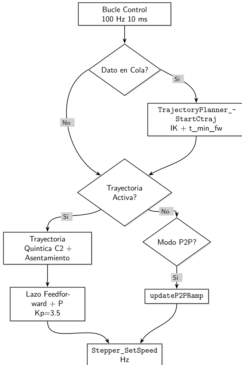
Figura 3.4: Diagrama de bloques Firmware Detalle 2: mControlTask y Planificador Quintico.
