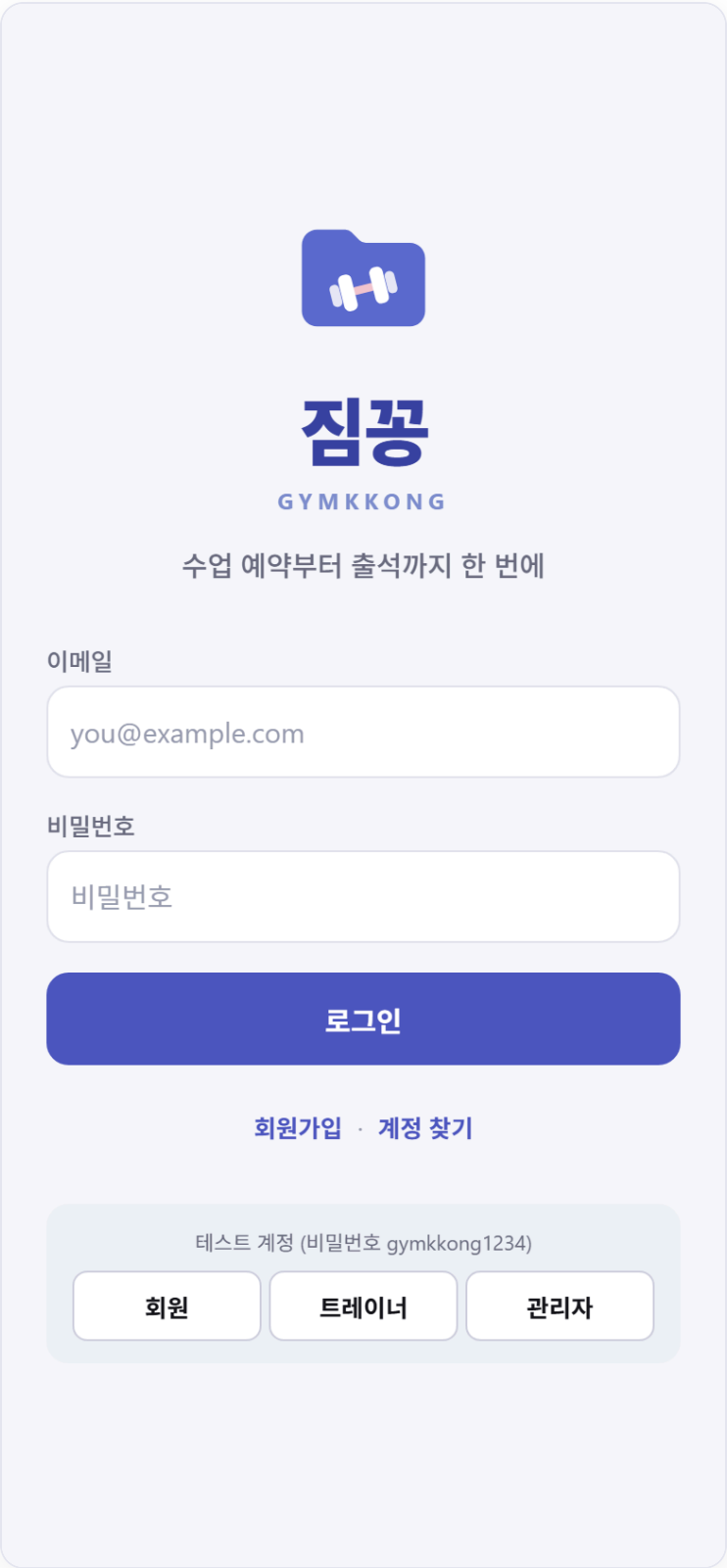
1 로그인 화면
