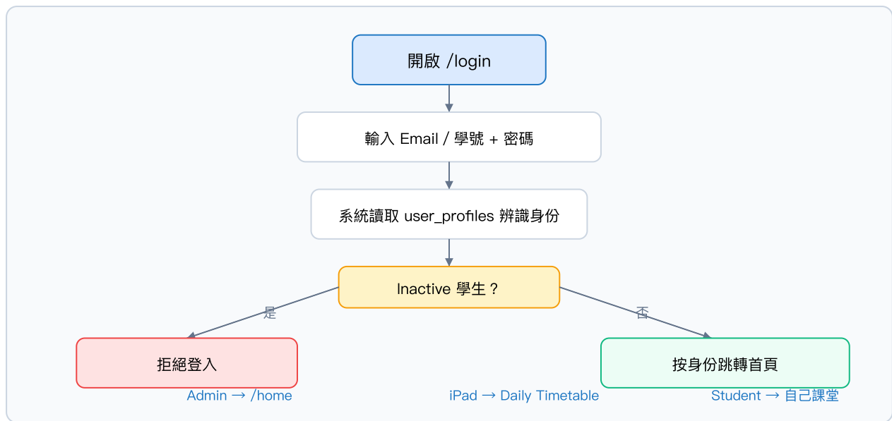
圖 2 — 登入流程
