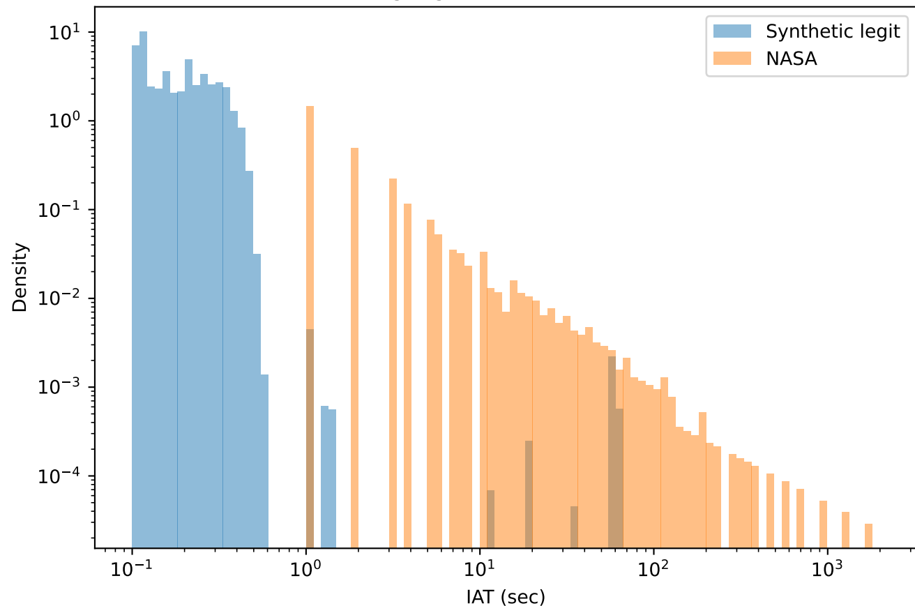
Log-log scale (KS=0.994)
