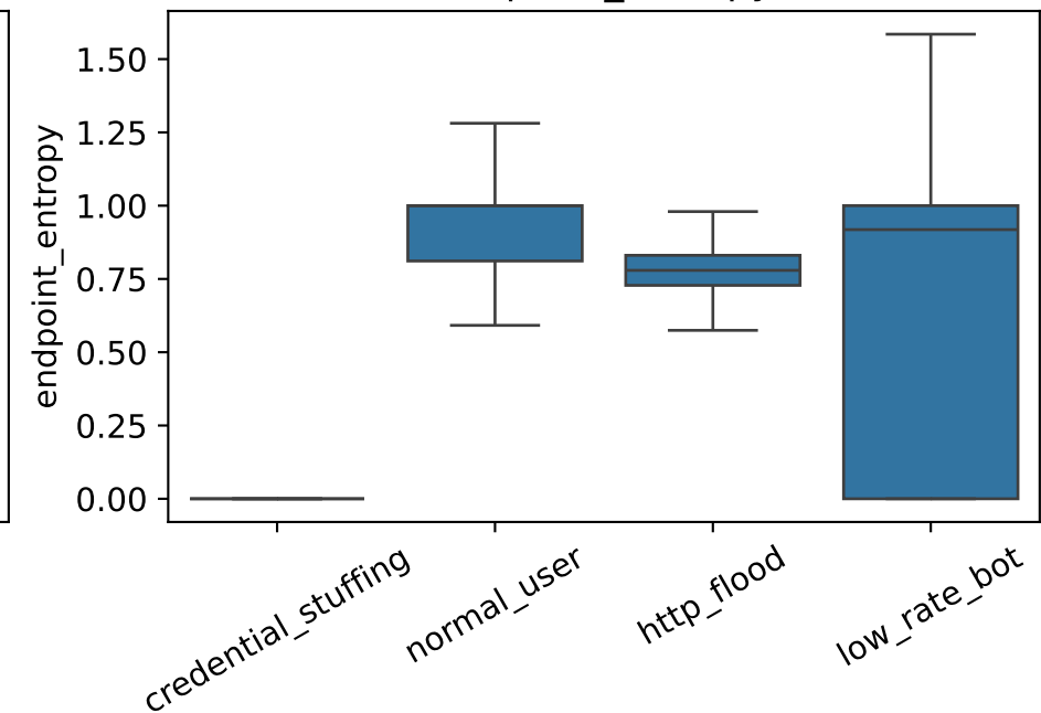
endpoint_entropy
