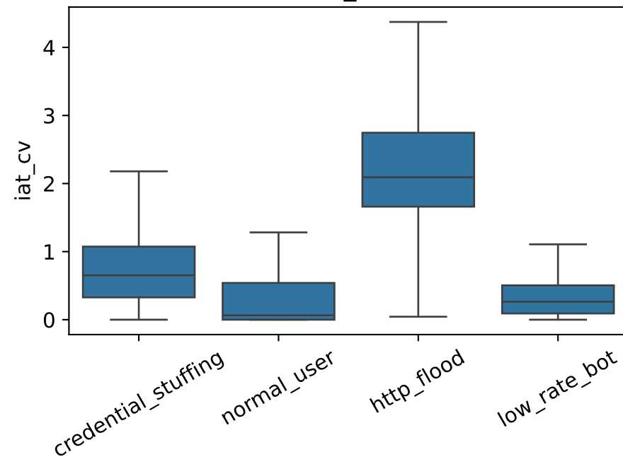
iat_cv
