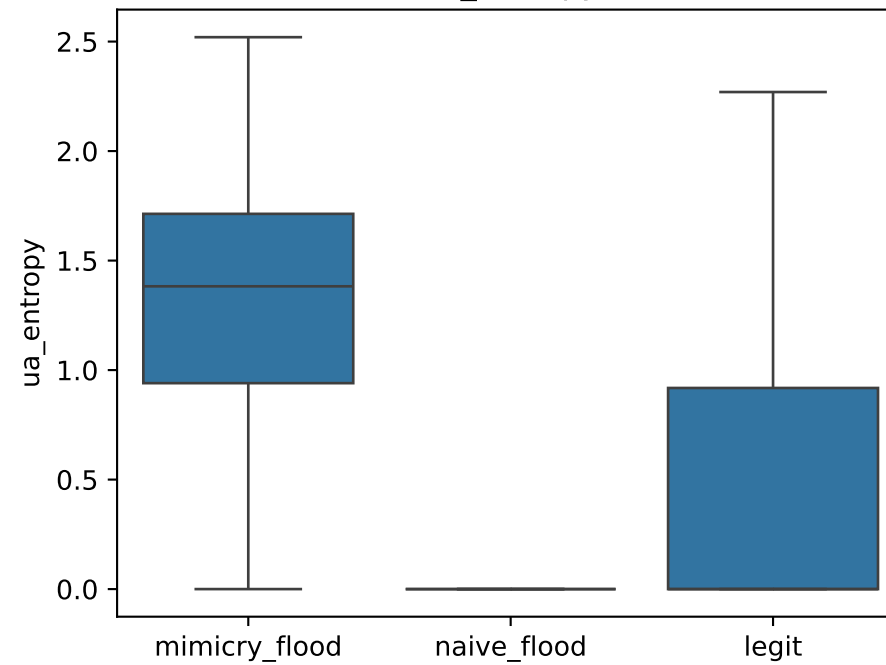
ua_entropy
