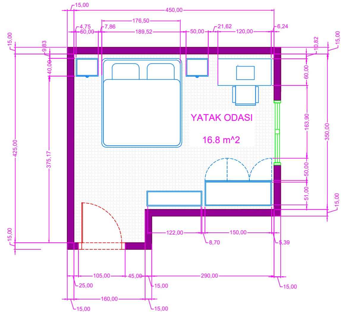
Ölçülendirilmiş Plan
