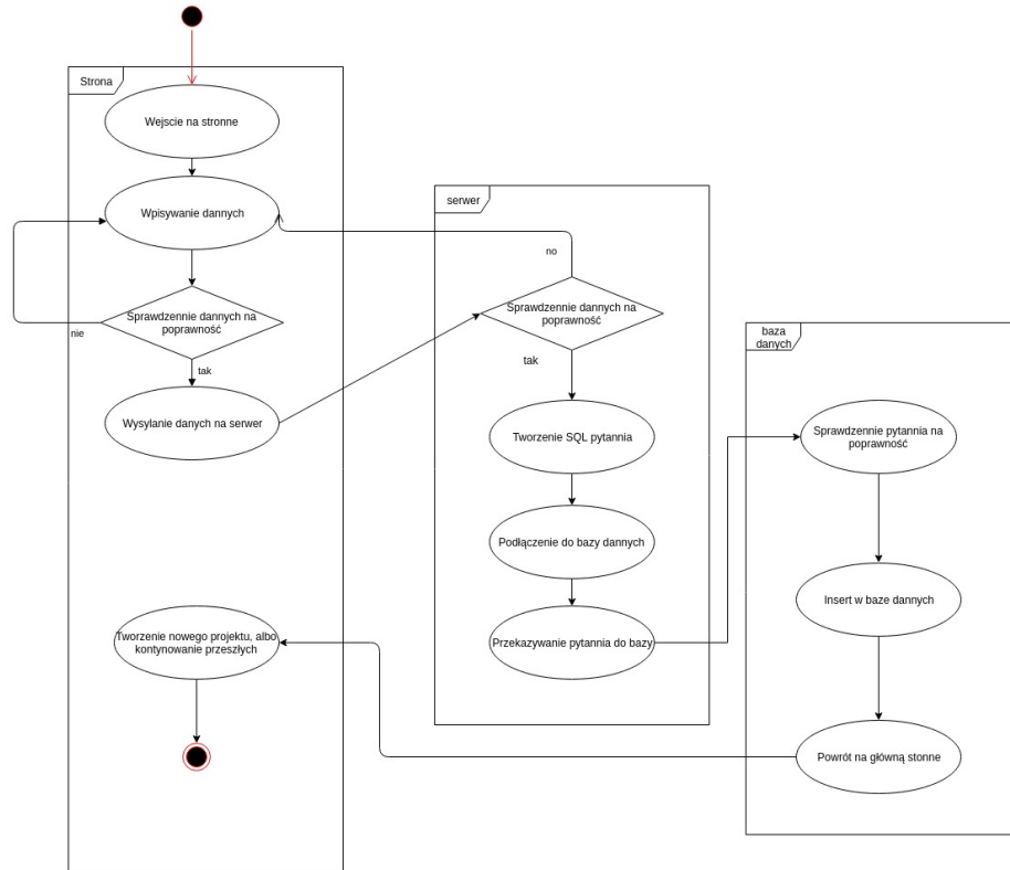
Diagram rejestracji użytkownika
