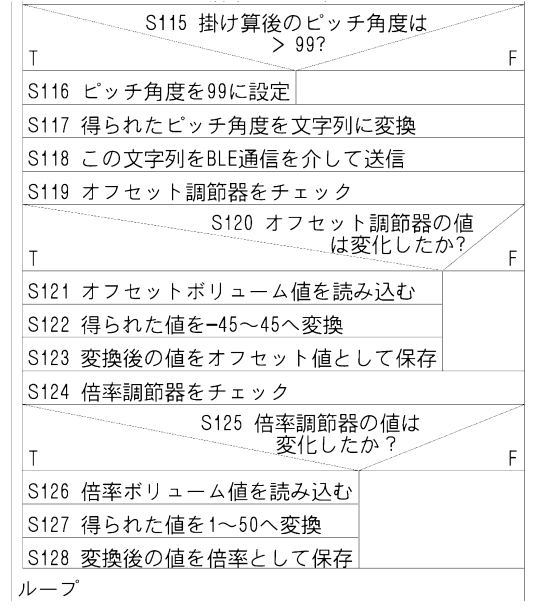
検出器側処理フローチャートII
