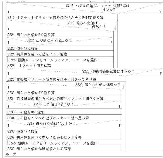
アクチュエータ側処理フローチャートII
