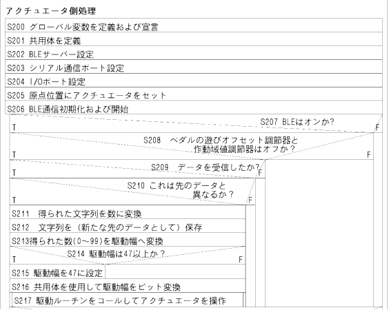
アクチュエータ側処理フローチャートI
