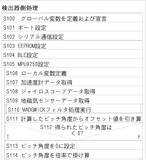
検出器側処理フローチャートI
