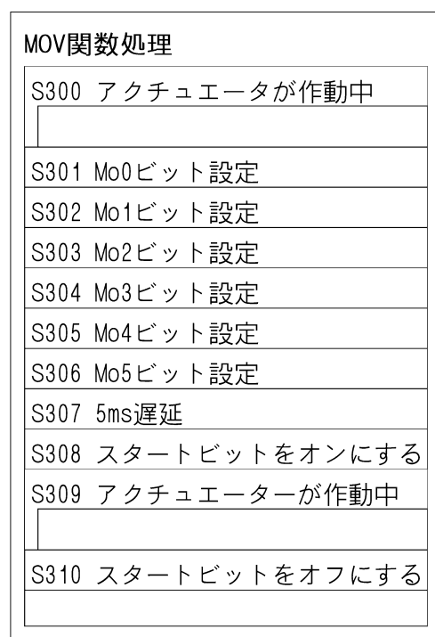
MOV関数フローチャート
