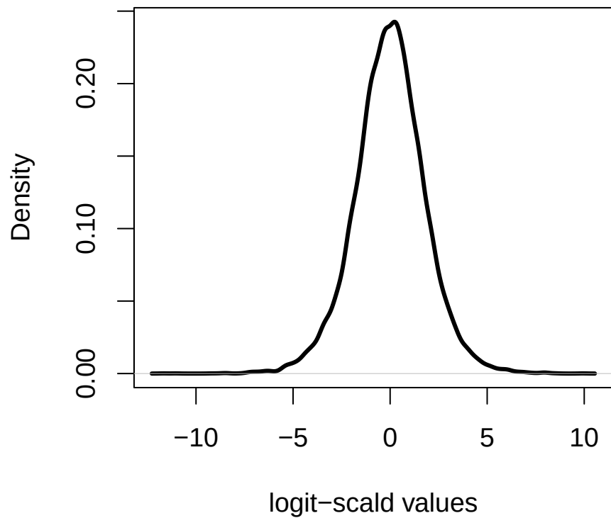
logit-scale
