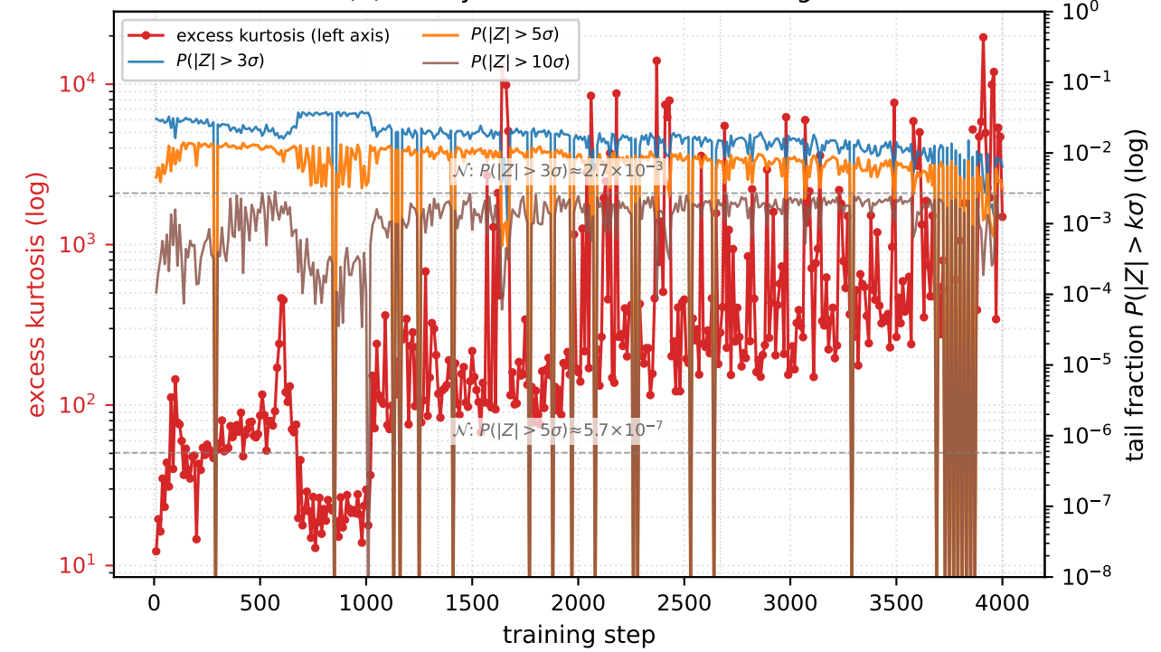
(d) Heavy-tail metrics over training
