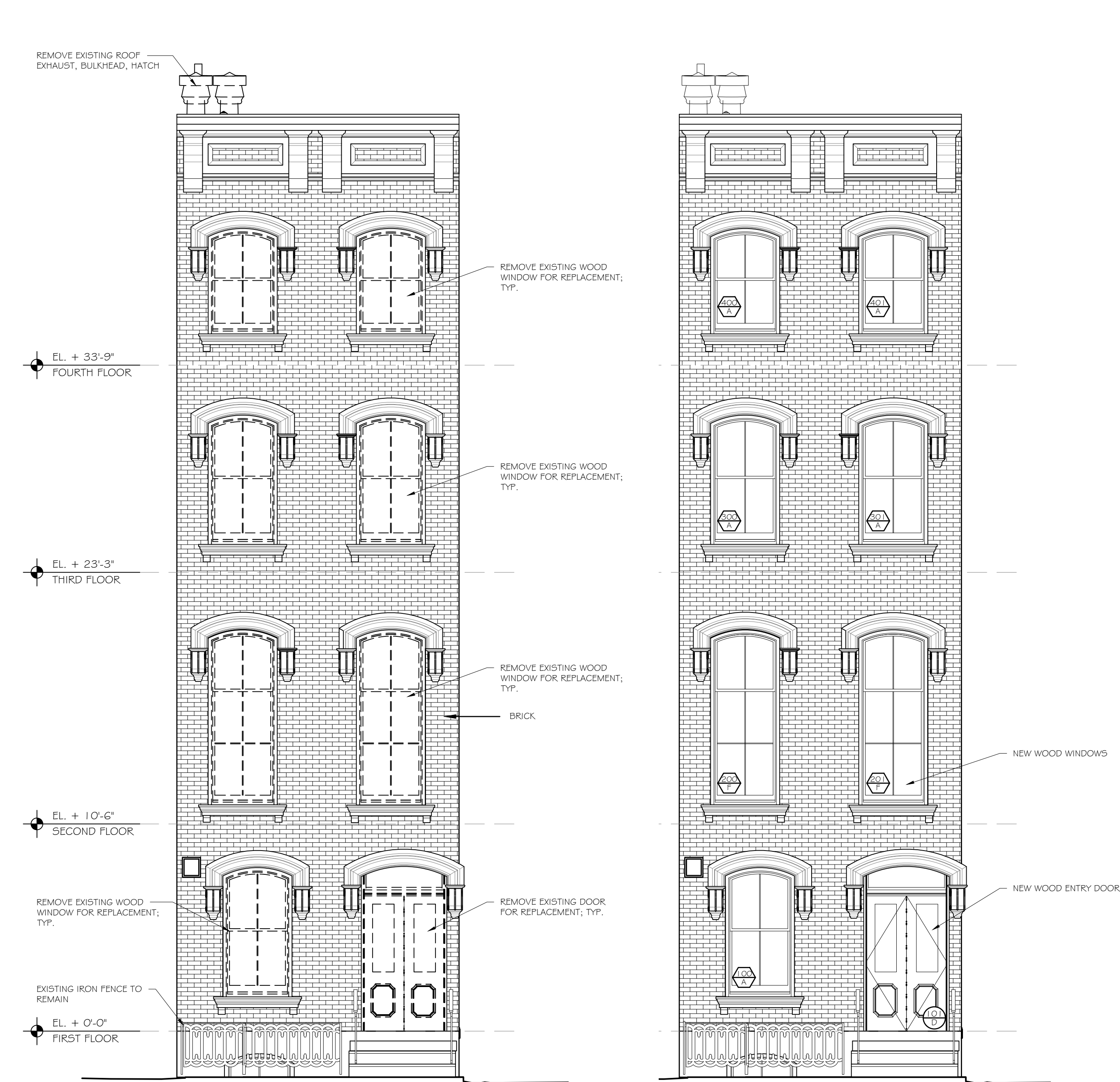
1 DEMO FRONT ELEVATION A-200 SCALE: 1/4"= 1'-0"
