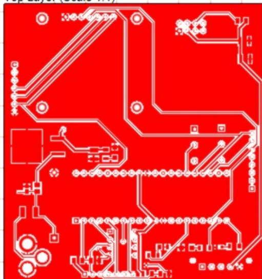
Top Layer (Scale 1:1)
