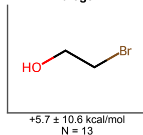
Halogen
