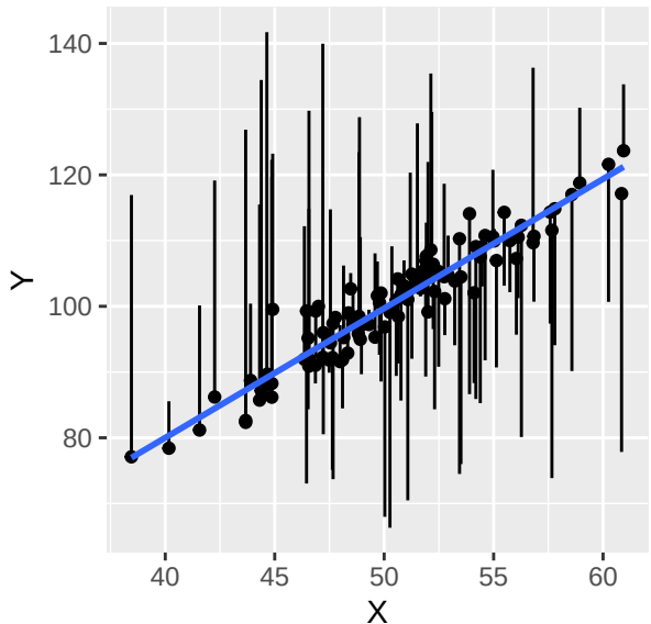
Heteroscedastic Data
