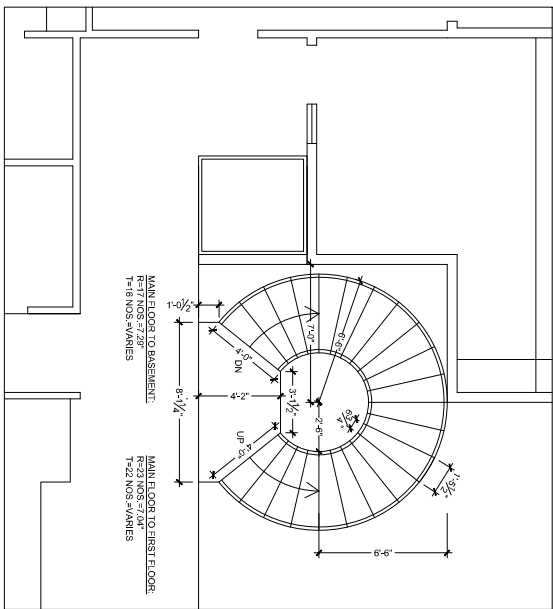
1 SPIRAL STAIR DETAIL A2 Scale: 1/8" = 1'-0"
