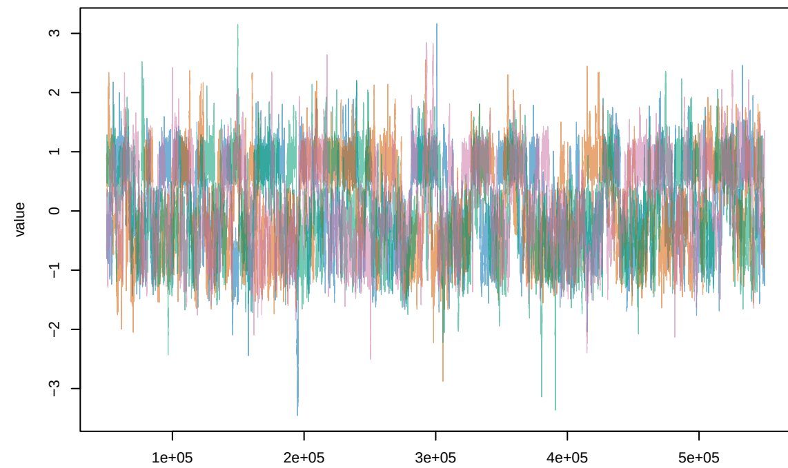
gamma_bio30
