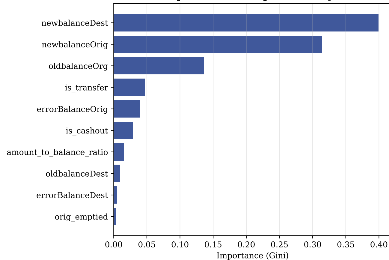
(d) Top-10 Feature Importance (Hybrid)
