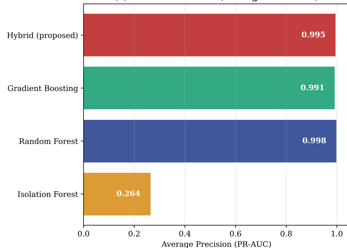
(b) Precision-Recall (Average Precision)
