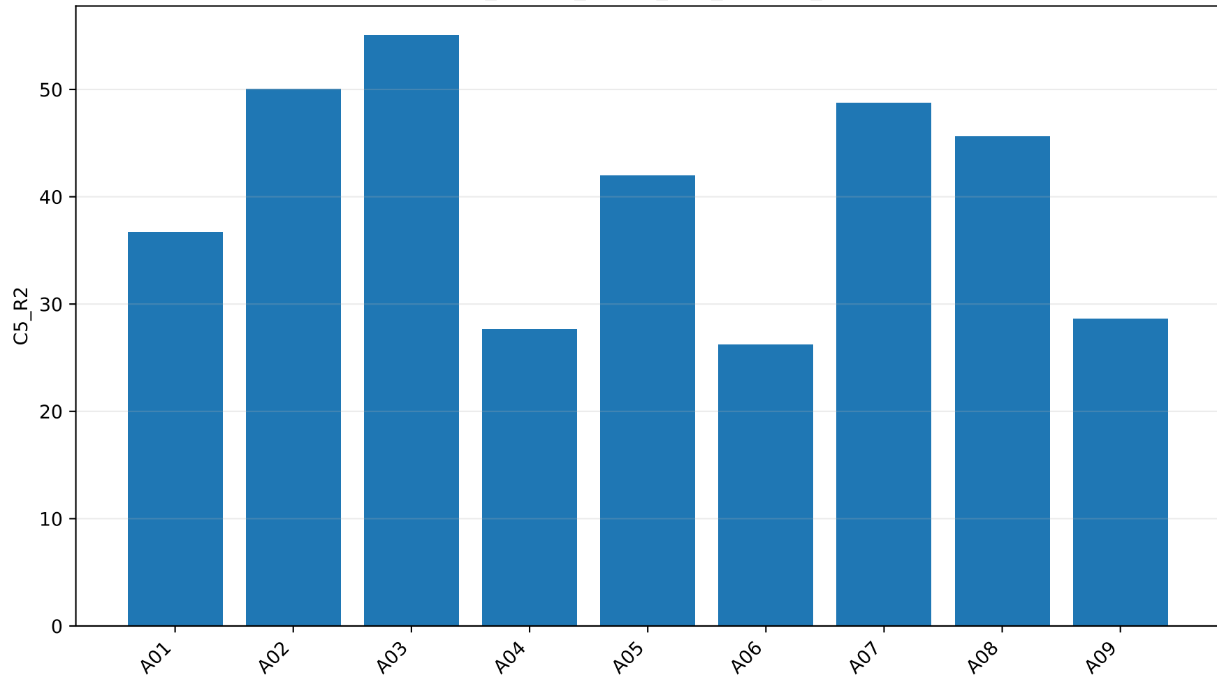
eog_central_region_A01_A09: C5_R2
