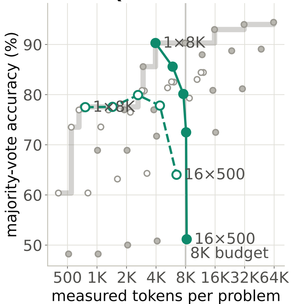
Qwen3-1.7B
