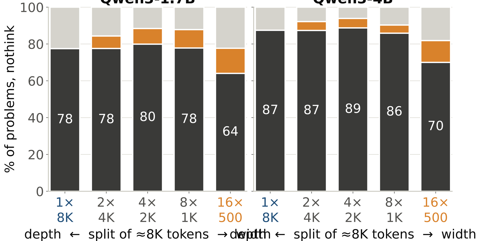
Qwen3-1.7B
